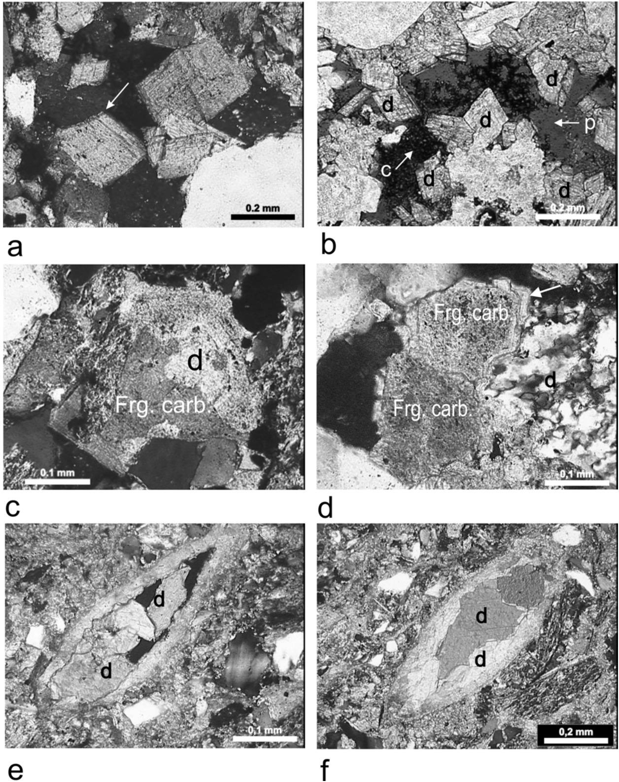
Figura 8 - Micrografias das lâminas petrográficas provenientes do Campo de Camorim (Bacia Sergipe-Alagoas) detalhando: dolomita em sela ( saddle dolomite ) caracterizada pelas faces curvas (nicóis cruzados). cimento de dolomita romboédrica nas bordas dos grãos, preenchendo parcialmente os poros intergranulares (p) com presença de caulinita (c) (nicóis paralelos). fragmento carbonático (frg. carb.) substituído por dolomita (nicóis cruzados). fragmento carbonático nucleando a precipitação do cimento dolomítico (seta) (nicóis cruzados). bioclasto com interior parcialmente recristalizado para dolomita (d) (nicóis cruzados). bioclasto completamente recristalizado para dolomita (d) (nicóis cruzados).
