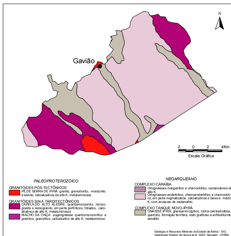
Figura 3 – Esboço geológico.
