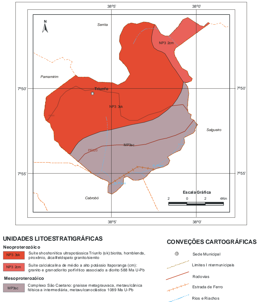
Figura 3- Mapa Geológico
