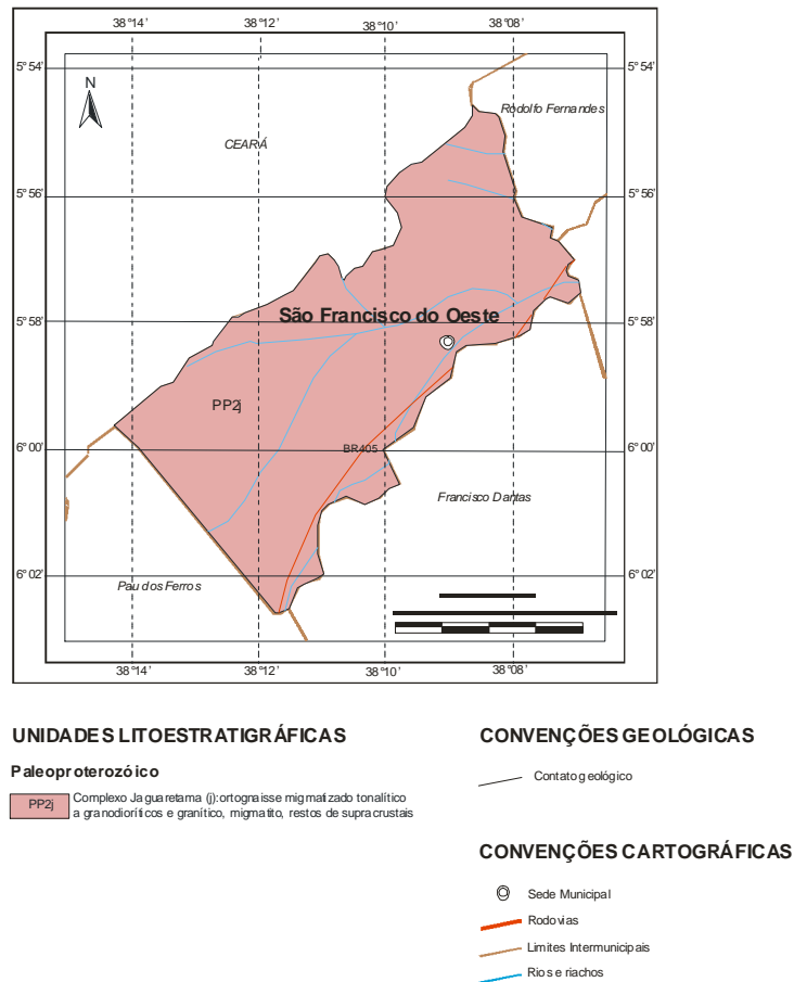
Figura 3 - Mapa Geológico
