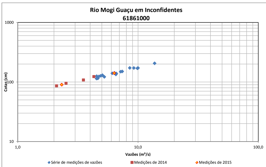
Figura 92 - Medições de descarga líquida do Rio Mogi Guaçu em Inconfidentes
