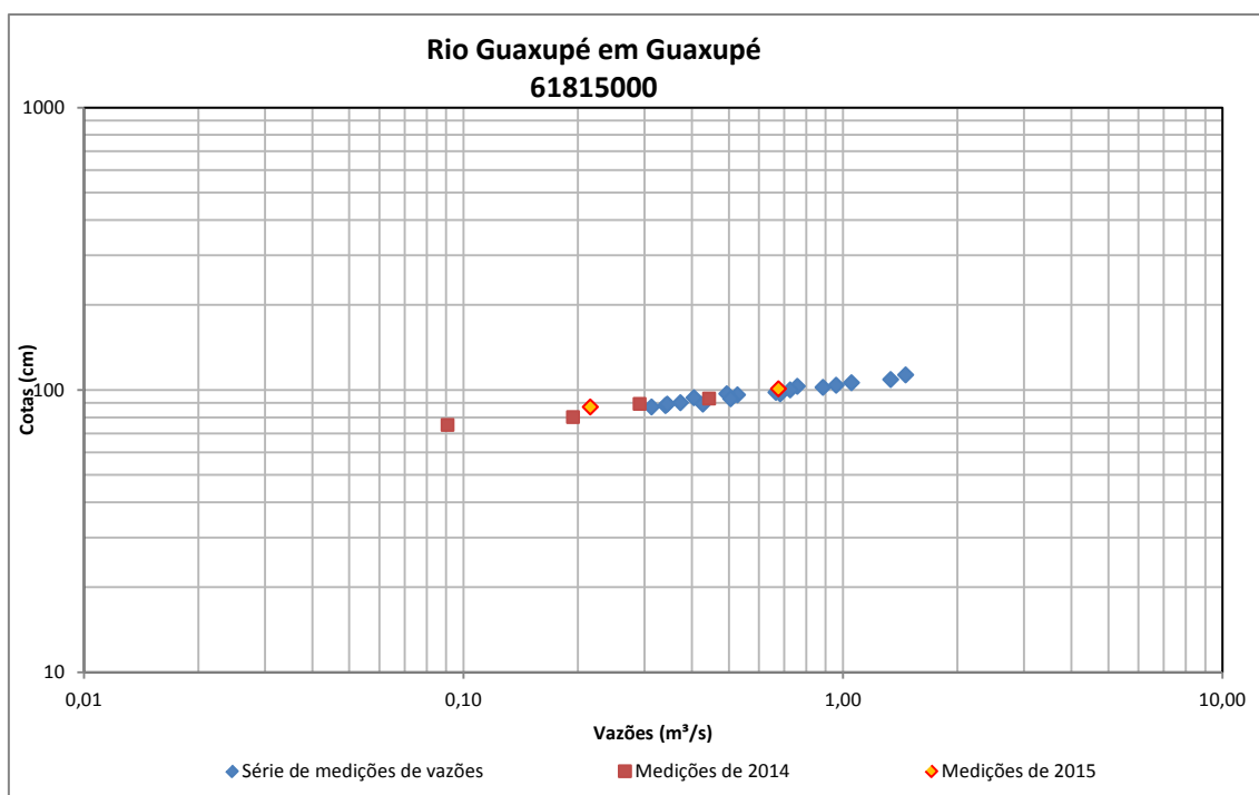
Figura 91 - Medições de descarga líquida do Rio Guaxupé em Guaxupé
