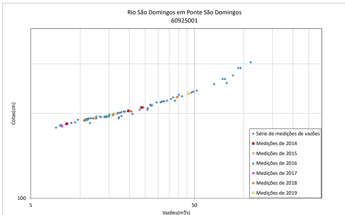
Figura 50 - Resumo de medições de descarga no rio São Domingos em Ponte São Domingos (60925001)
