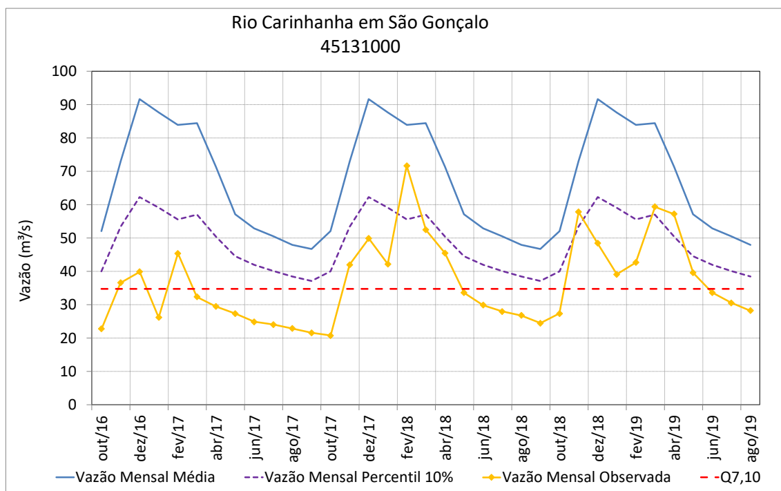
Figura 75 – Vazões médias mensais do rio Carinhanha em São Gonçalo
