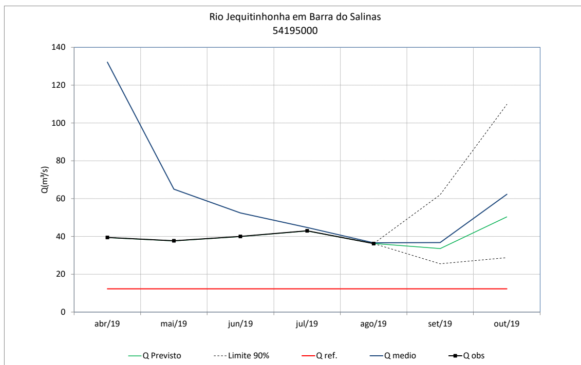
Figura 77 – Previsão de vazões do rio Jequitinhonha em Barra do Salinas
