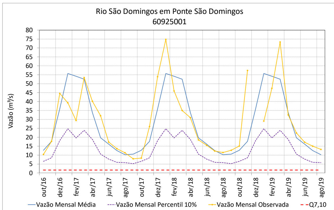
Figura 93 – Vazões médias mensais do rio São Domingos em Ponte São Domingos
