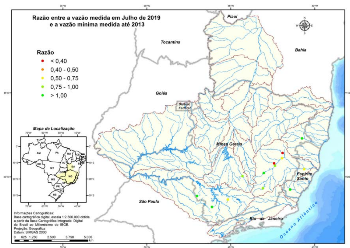
Figura 20 - Razão entre a vazão medida em julho de 2019 e a vazão mínima medida até 2013.
