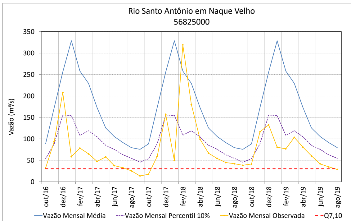
Figura 84 – Vazões médias mensais do rio Santo Antônio em Naque Velho
