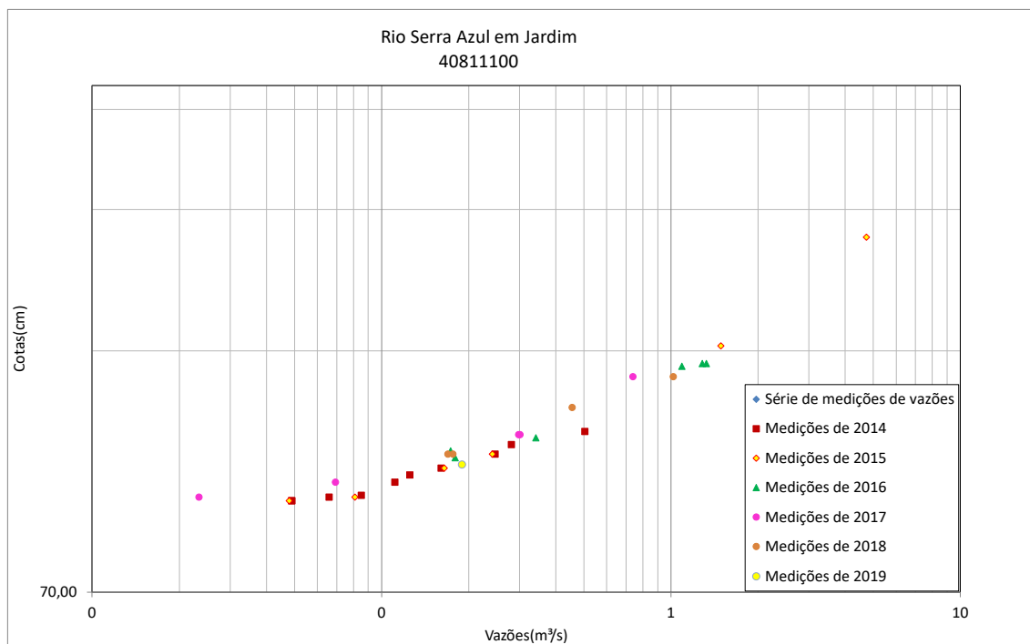
Figura 25 - Resumo de medições de descarga no rio Serra Azul em Jardim (40811100)
