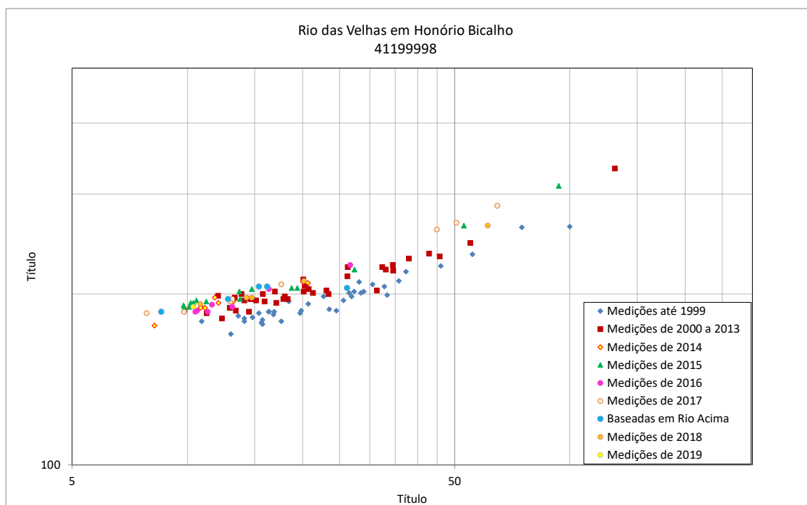
Figura 27 - Resumo de medições de descarga no rio das Velhas em Honório Bicalho (41199998)
