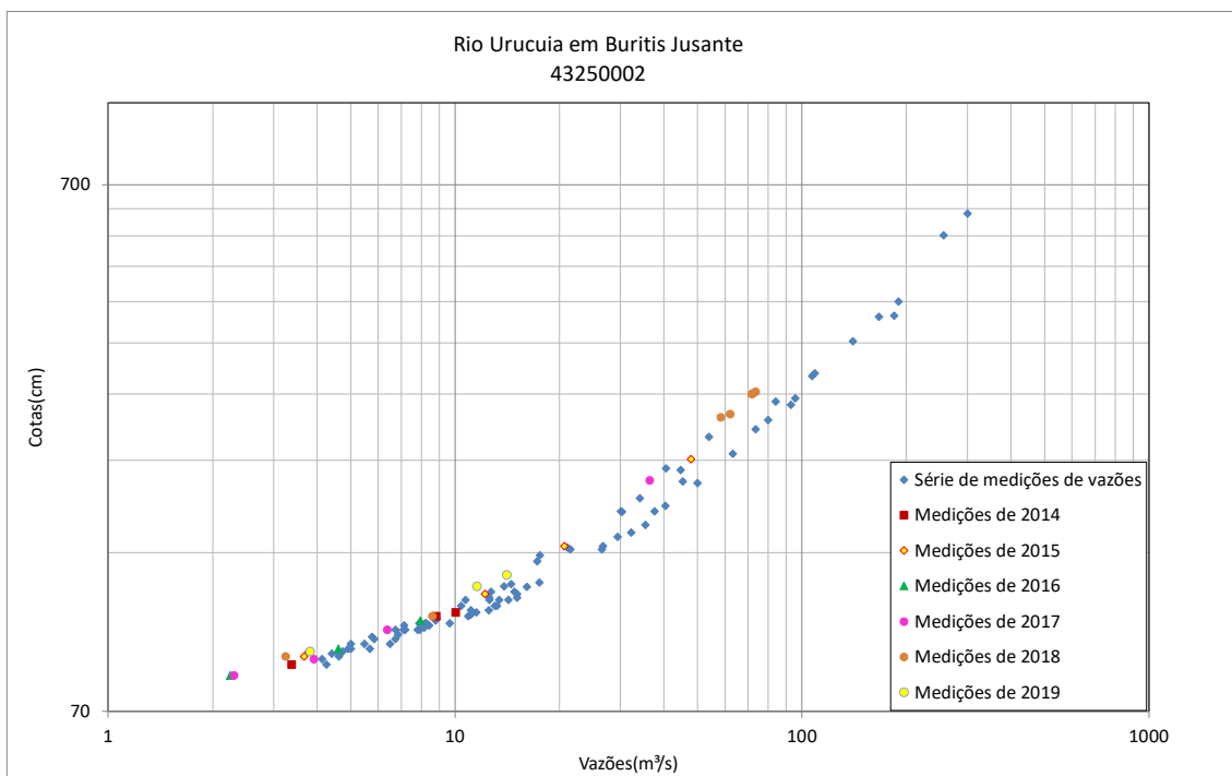
Figura 32 - Resumo de medições de descarga no rio Urucuia em Buritis Jusante (43250002)
