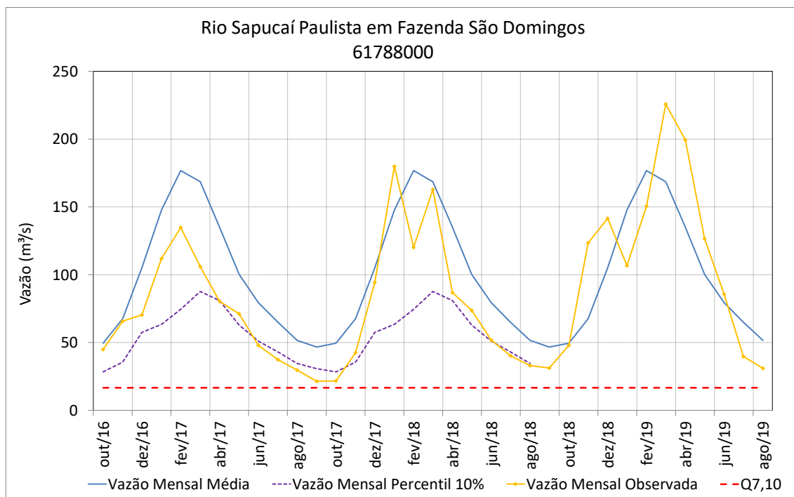
Figura 97 – Vazões médias mensais do rio Sapucaí Paulista em Fazenda São Domingos
