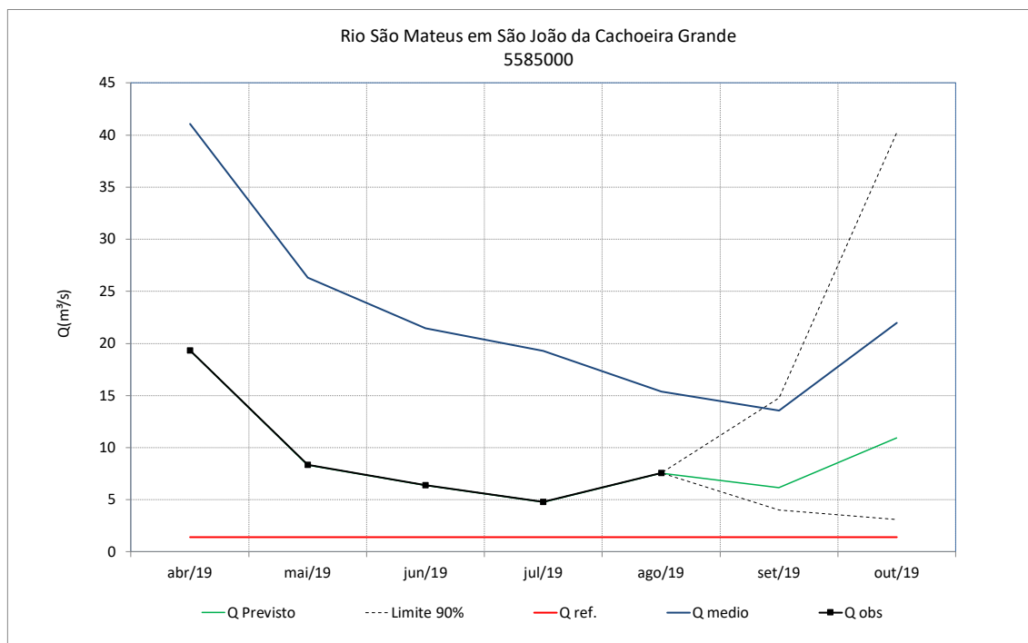
Figura 80 – Previsão de vazões do rio São Mateus em São João da Cachoeira Grande
