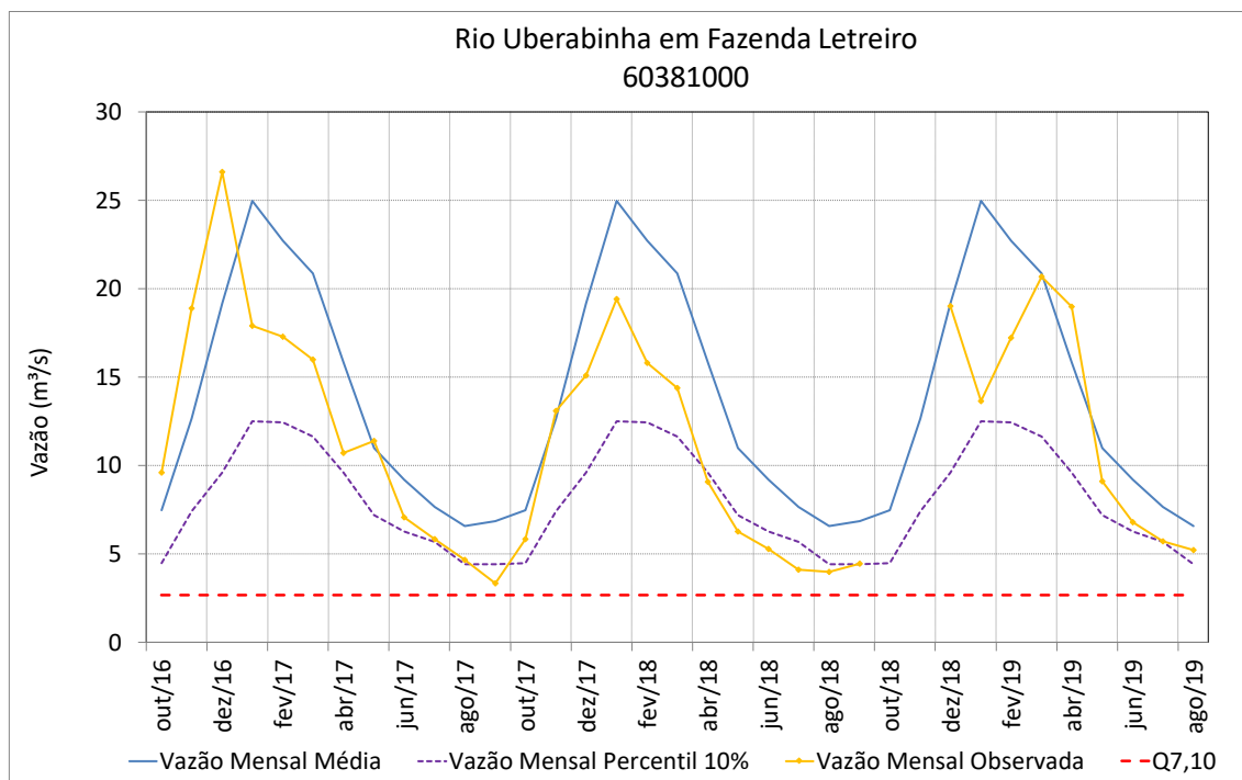
Figura 91 – Vazões médias mensais do rio Uberabinha em Fazenda Letreiro
