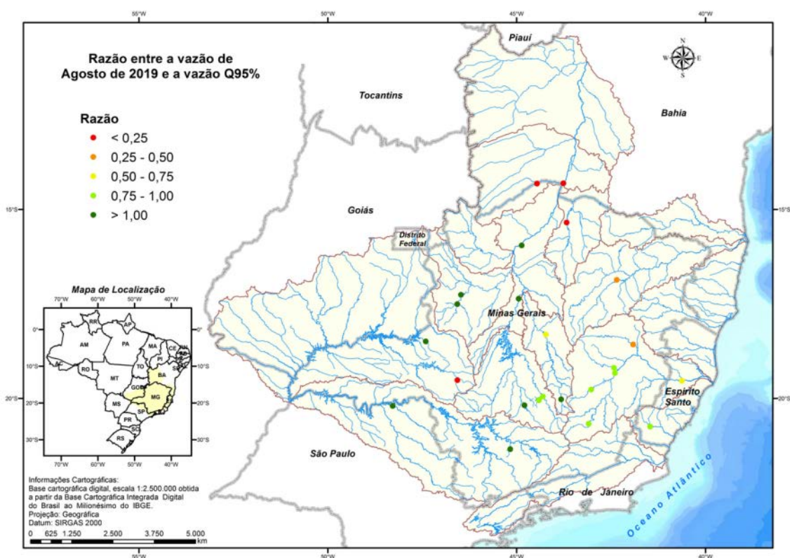
Figura 18 - Razão entre a vazão de agosto de 2019 e a vazão Q_{95\%} .
