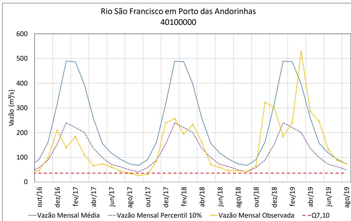
Figura 64 – Vazões médias mensais do rio São Francisco em Porto das Andorinhas
