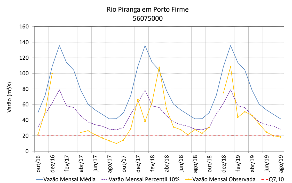
Figura 81 – Vazões médias mensais do rio Piranga em Porto Firme
