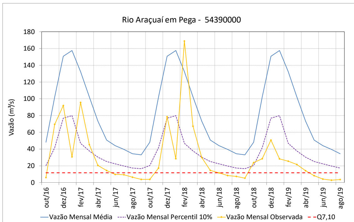
Figura 78 – Vazões médias mensais do rio Araçuai em Pega
