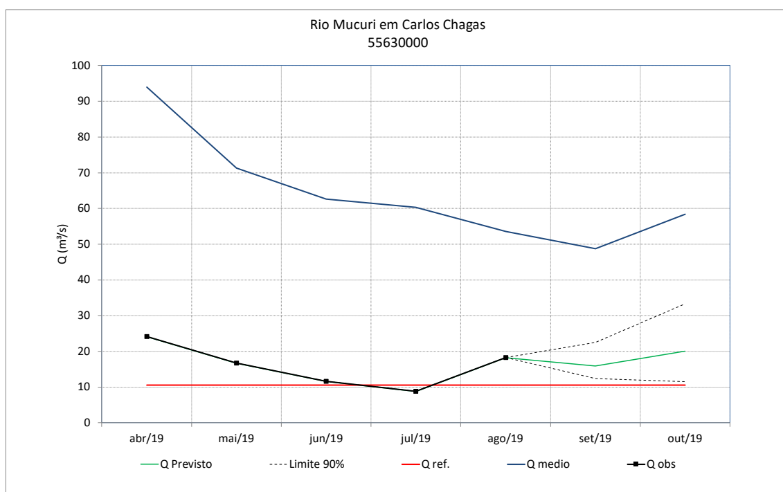
Figura 79 - Previsão de vazões do rio Mucuri em Carlos Chagas
