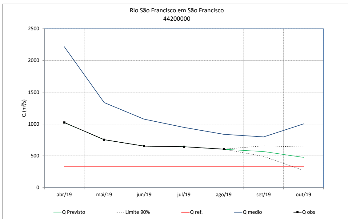
Figura 74 – Previsão de vazões do rio São Francisco em São Francisco
