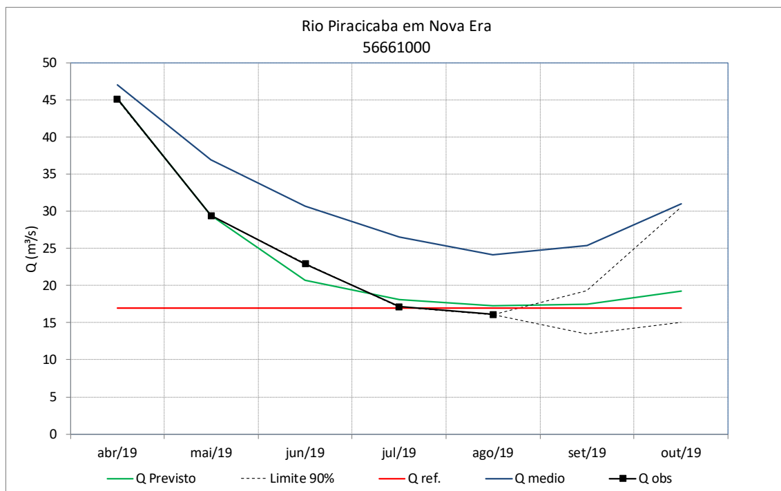
Figura 59 - Previsão de vazões do rio Piracicaba em Nova Era
