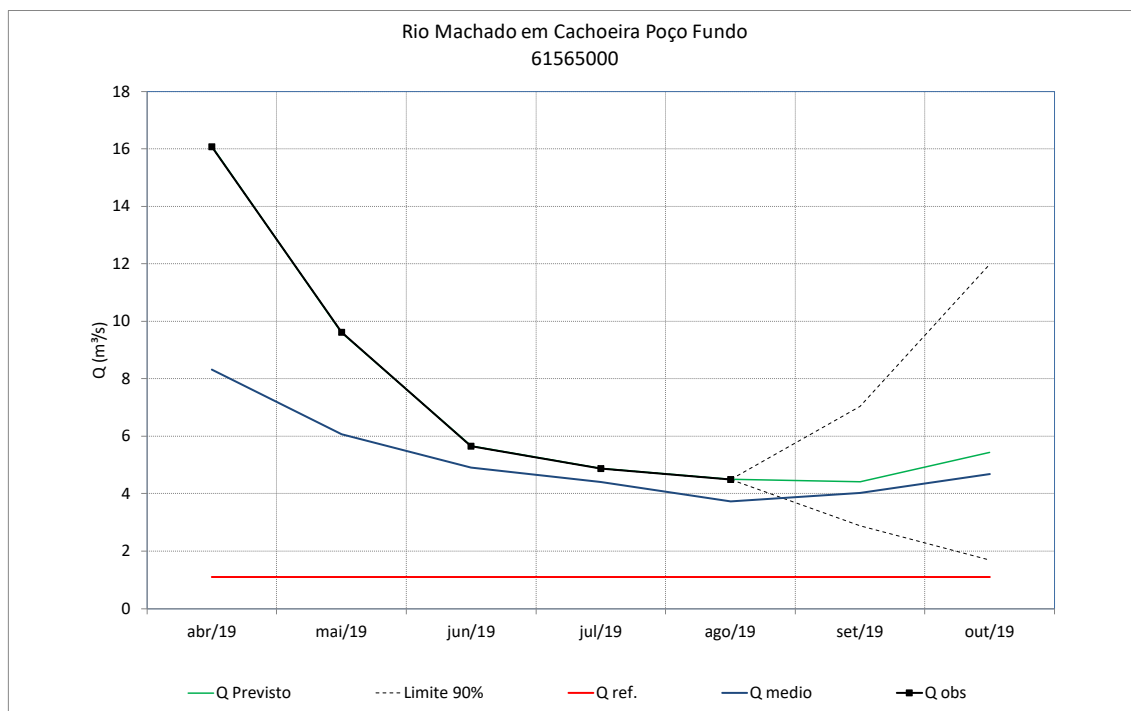
Figura 95 – Previsão de vazões do rio Machado em Cachoeira Poço Fundo
