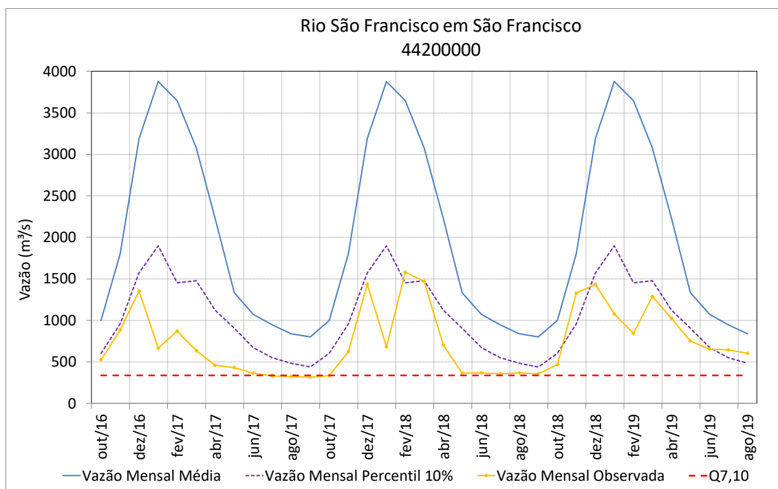
Figura 74 – Vazões médias mensais do rio São Francisco em São Francisco
