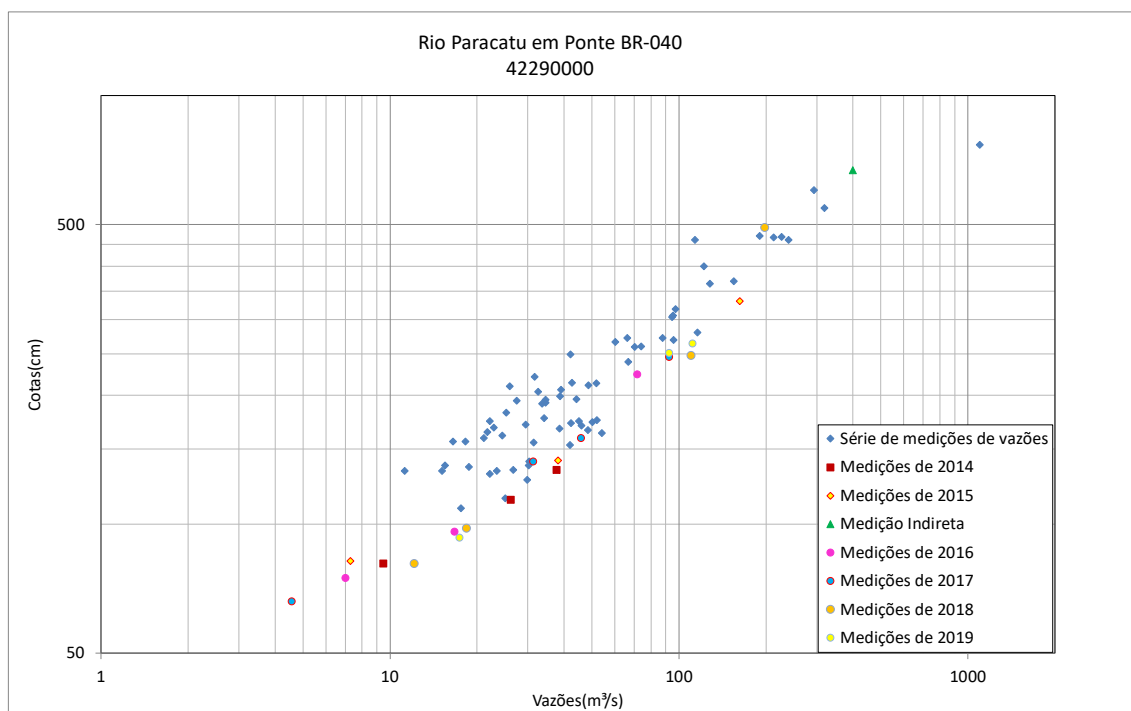
Figura 29 - Resumo de medições de descarga no rio Paracatu em Ponte BR-040 Paracatu (42290000)
