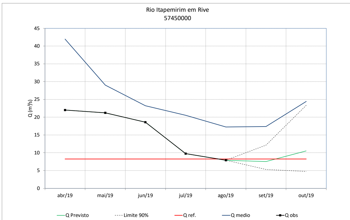
Figura 88 – Previsão de vazões do rio Itapemirim em Rive
