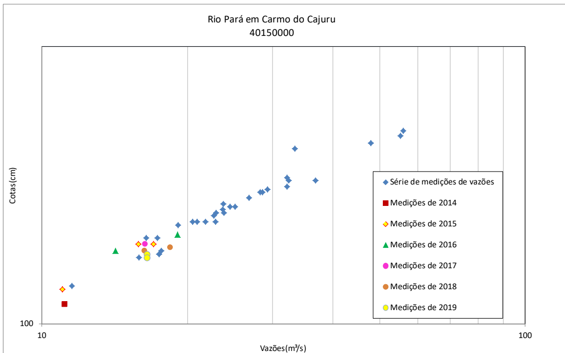
Figura 23 - Resumo de medições de descarga no rio Pará em Carmo do Cajuru (40150000)
