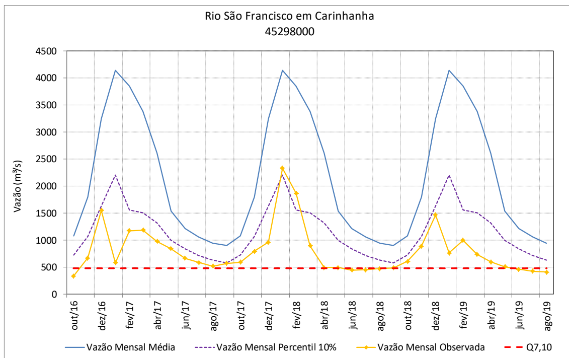
Figura 76 – Vazões médias mensais do rio São Francisco em Carinhanha
