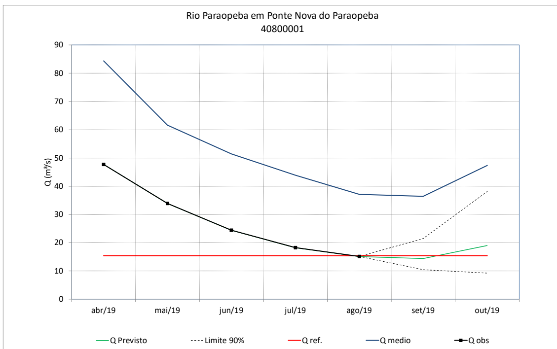
Figura 66 – Previsão de vazões do rio Paraopeba em Ponte Nova do Paraopeba
