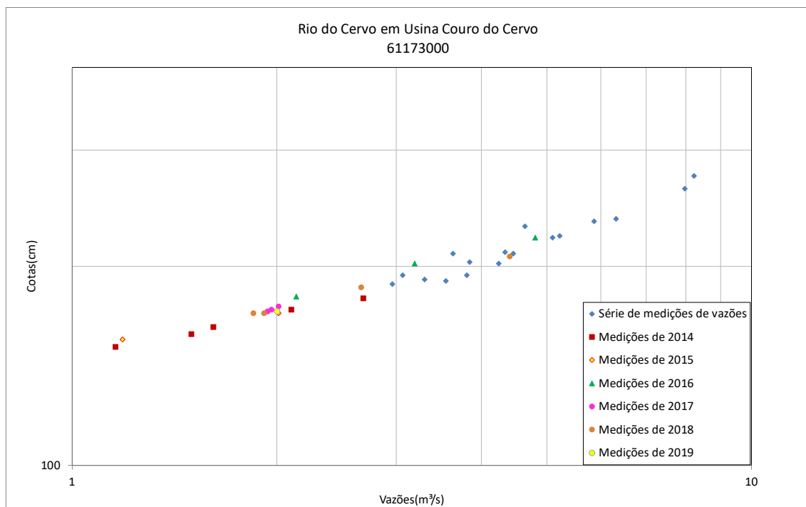
Figura 51 - Resumo de medições de descarga no rio Cervo em Usina Couro do Cervo (61173000)
