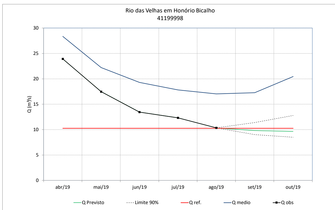
Figura 69 – Previsão de vazões do rio das Velhas em Honório Bicalho
