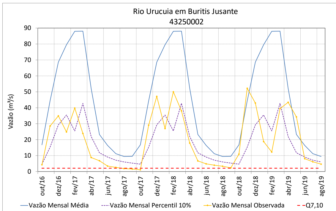
Figura 73 – Vazões médias mensais do rio Urucua em Buritis Jusante
