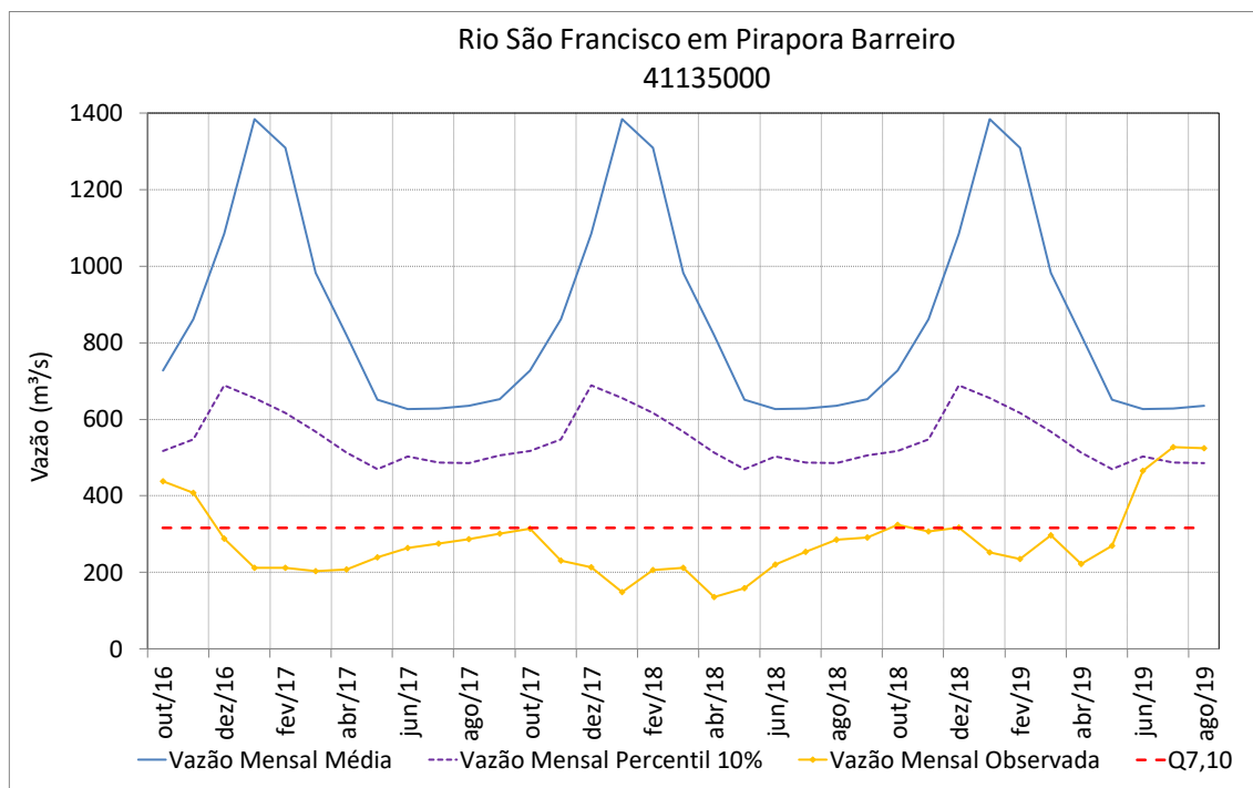
Figura 68 – Vazões médias mensais do rio São Francisco em Pirapora Barreiro
