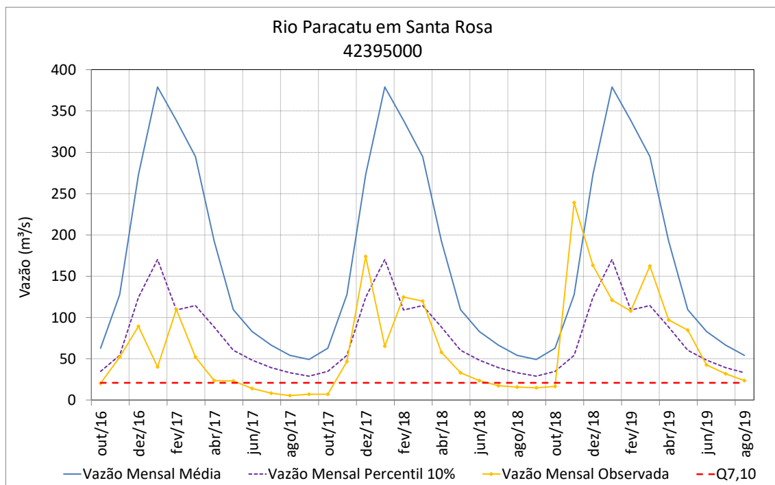
Figura 71 – Vazões médias mensais do rio Paracatu em Santa Rosa
