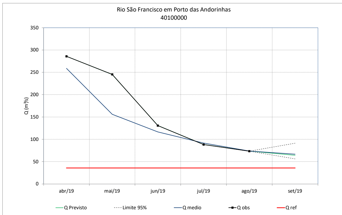
Figura 64 – Previsão de vazões do rio São Francisco em Porto das Andorinhas
