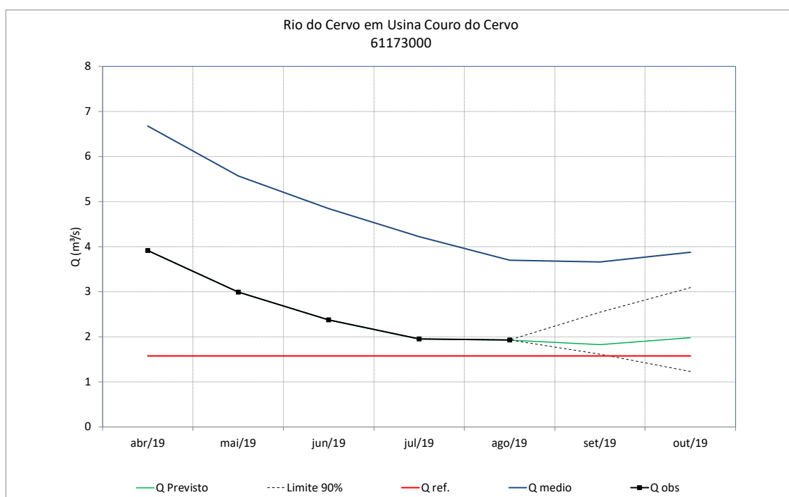
Figura 94 – Previsão de vazões do rio do Cervo em Usina Couro do Cervo
