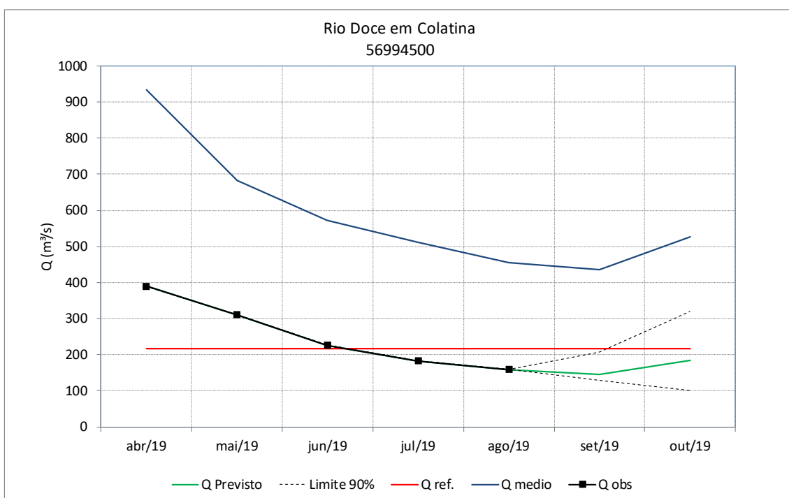
Figura 87 – Previsão de vazões do rio Doce em Colatina
