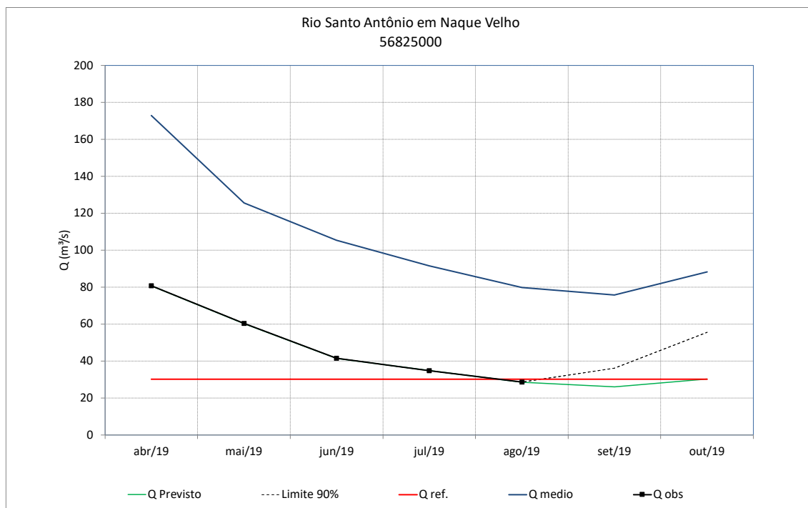
Figura 84 – Previsão de vazões do rio Santo Antônio em Naque Velho
