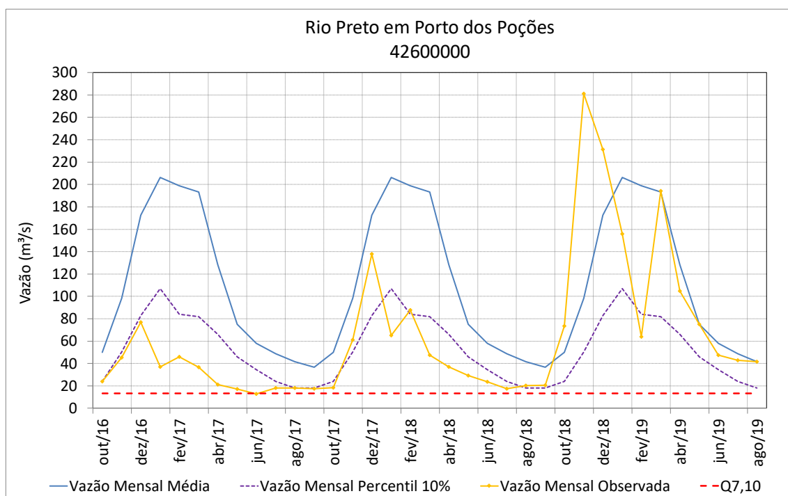
Figura 72 – Vazões médias mensais do rio Preto em Porto dos Poções
