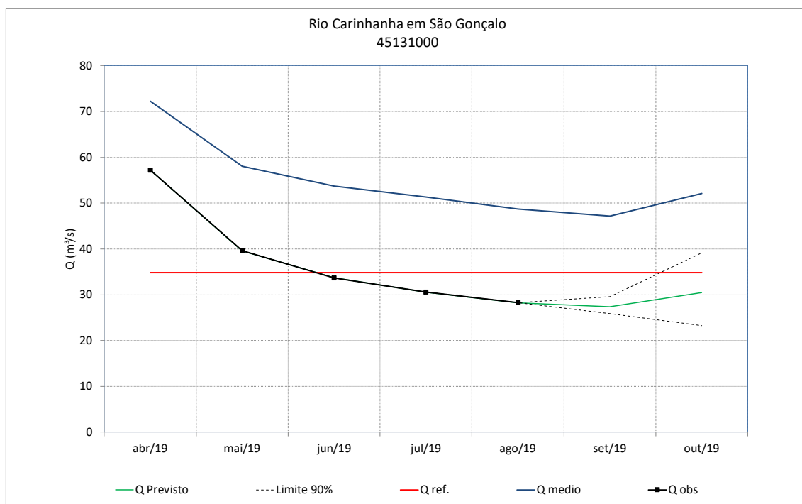
Figura 75 – Previsão de vazões do rio Carinhonha em São Gonçalo
