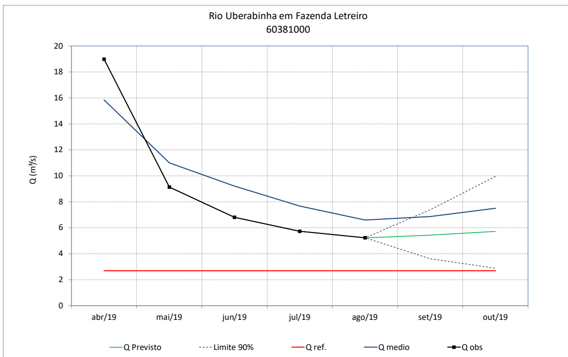
Figura 91 – Previsão de vazões do rio Uberabinha em Fazenda Letreiro
