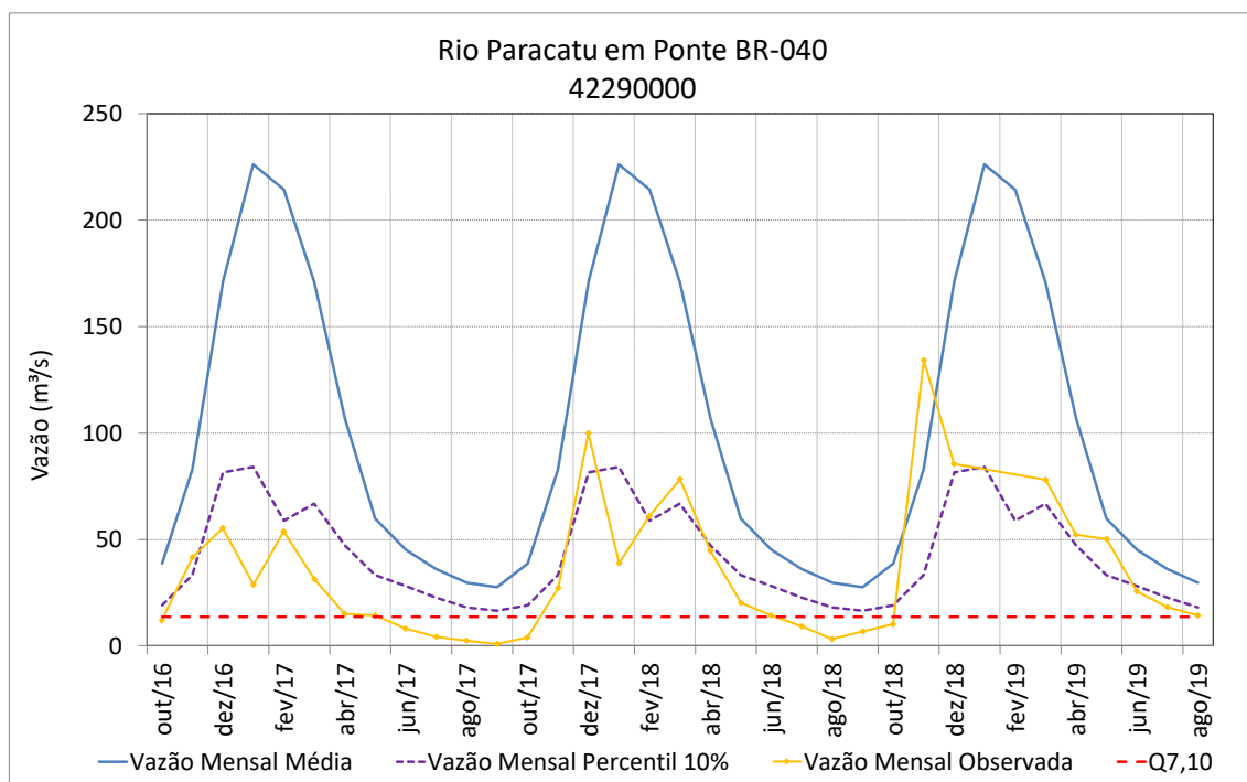
Figura 71 – Vazões médias mensais do rio Paracatu em Ponte BR-040
