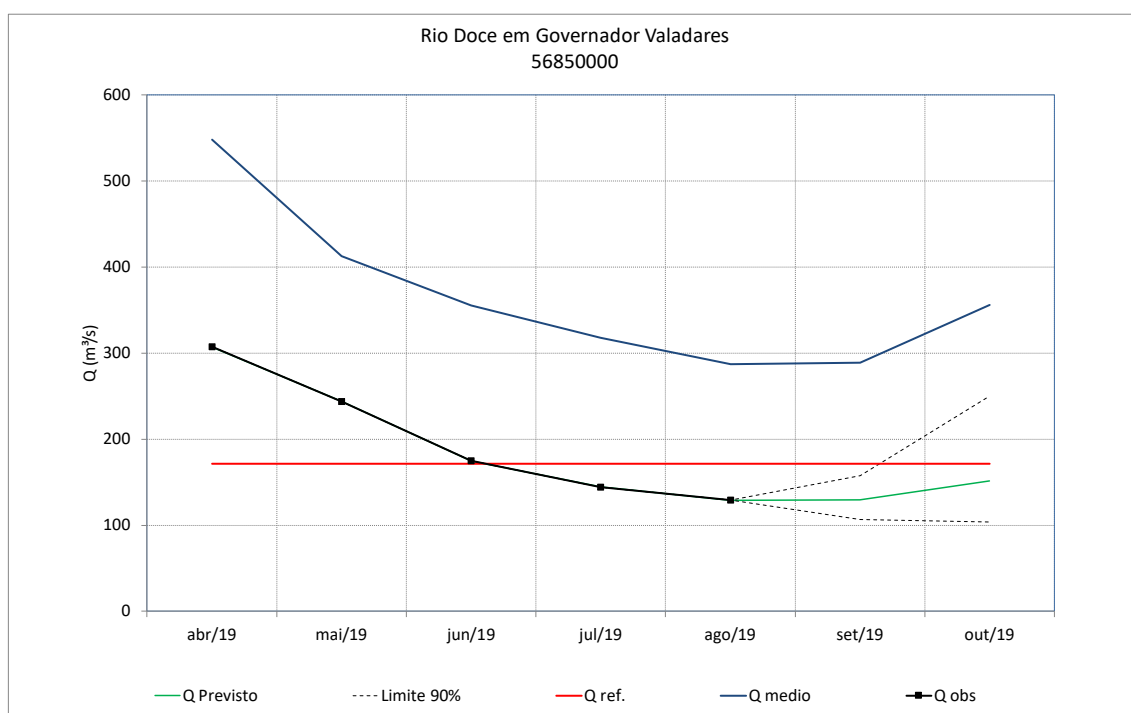
Figura 85 – Previsão de vazões do rio Doce em Governador Valadares
