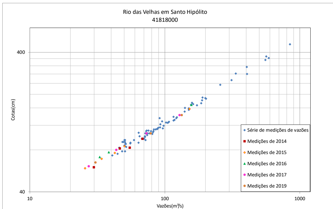
Figura 28 - Resumo de medições de descarga no rio das Velhas em Santo Hipólito (41818000)
