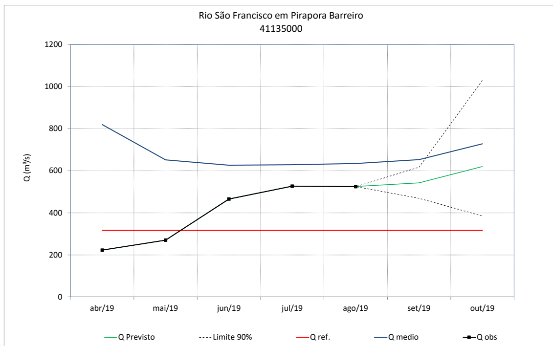
Figura 68 – Previsão de vazões do rio São Francisco em Pirapora Barreiro
