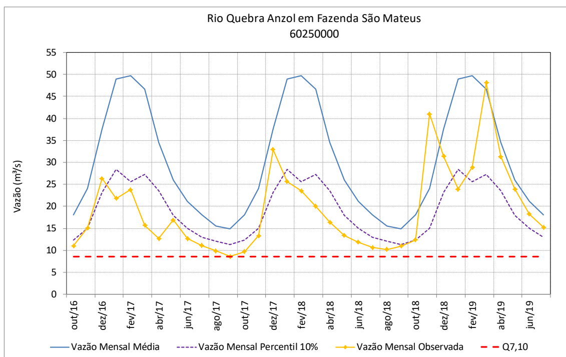
Figura 90 – Vazões médias mensais do rio Quebra Anzol em Fazenda São Mateus
