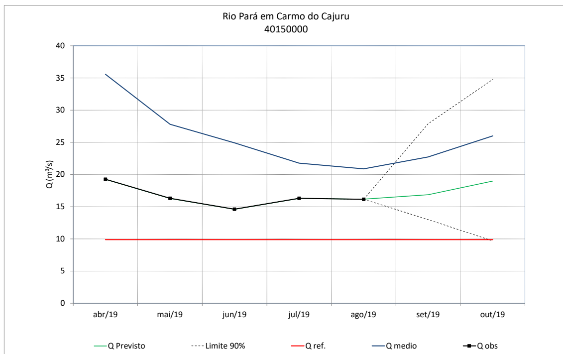
Figura 58 - Previsão de vazões do rio Pará em Carmo do Cajuru
