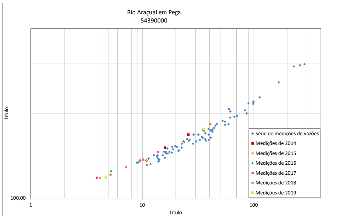
Figura 37 - Resumo de medições de descarga no rio Araçuai em Pega (54390000)
