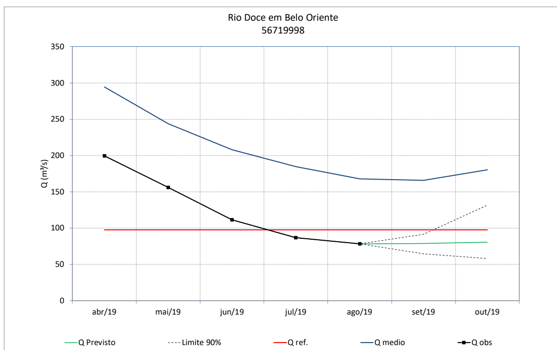
Figura 60 – Previsão de vazões do rio Doce em Belo Oriente
