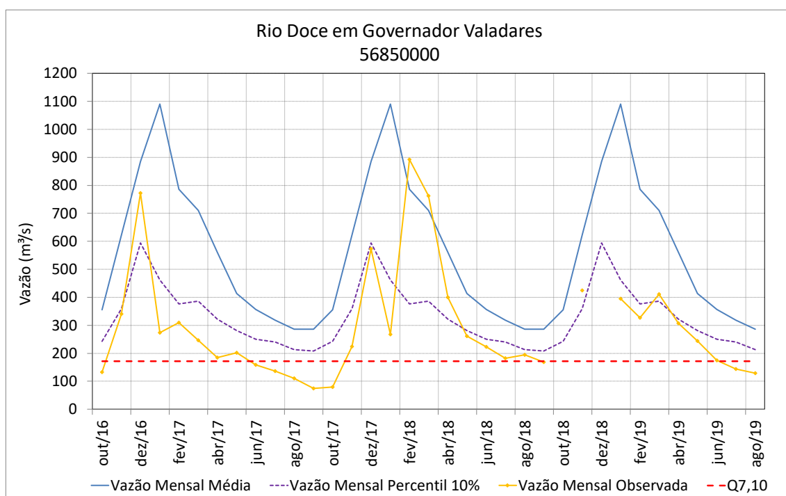
Figura 85 – Vazões médias mensais do rio Doce em Governador Valadares
