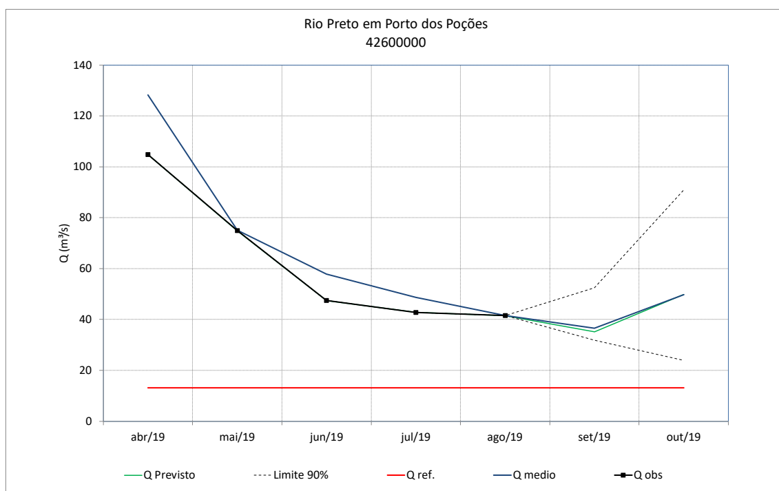
Figura 72 – Previsão de vazões do rio Preto em Porto dos Poções
