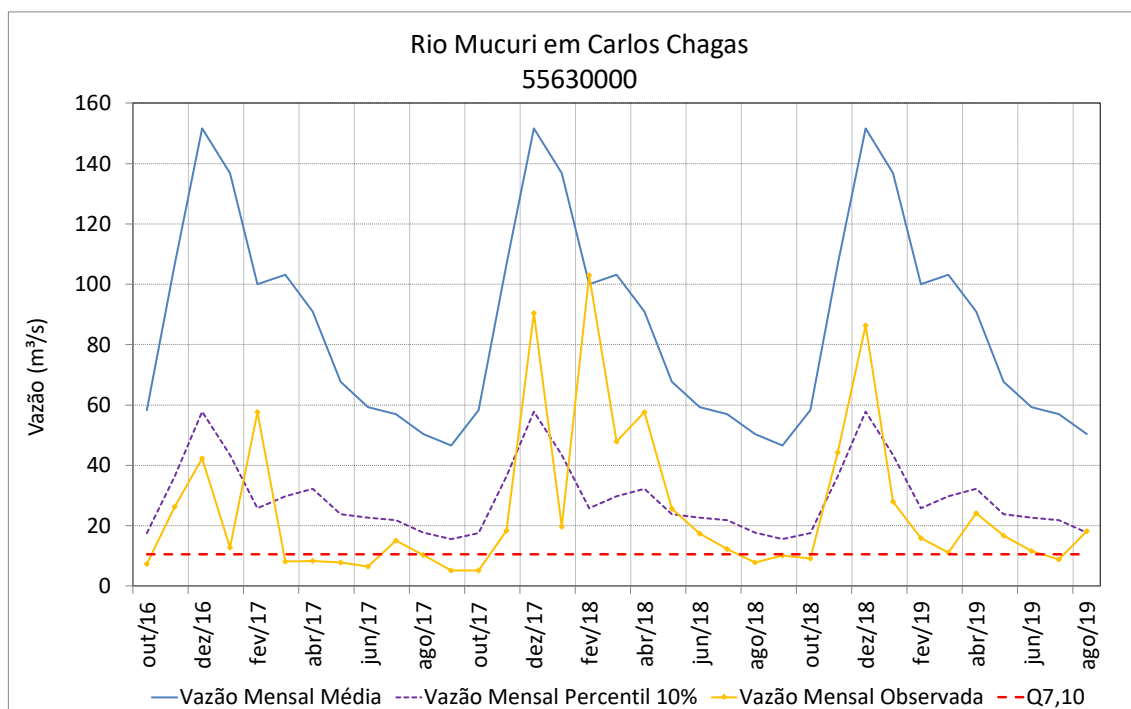
Figura 79 - Vazões médias mensais do rio Mucuri em Carlos Chagas
