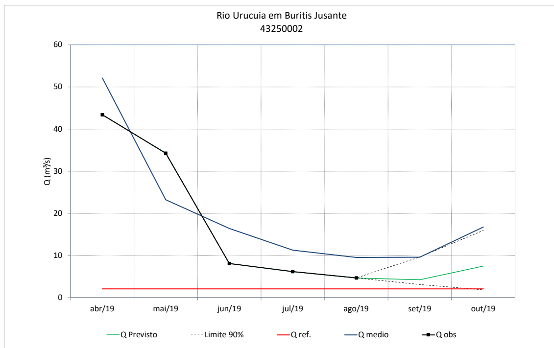
Figura 73 – Previsão de vazões do rio Urucuia em Buritis Jusante
