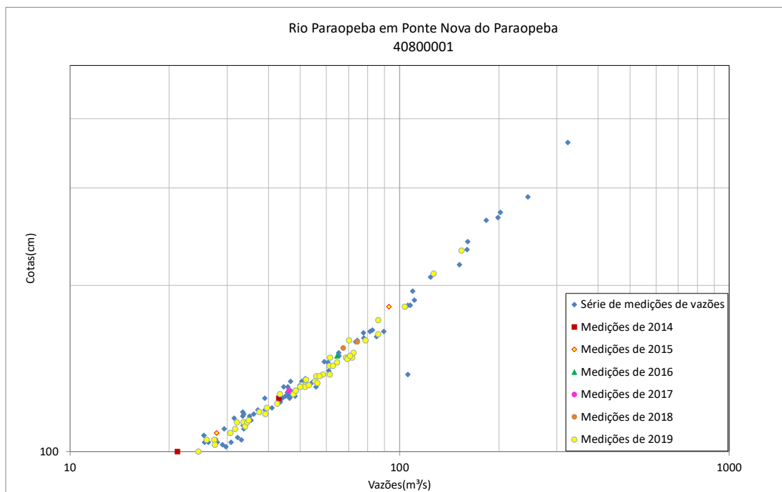
Figura 24 - Resumo de medições de descarga no rio Paraopeba em Ponte Nova do Paraopeba (40800001)
