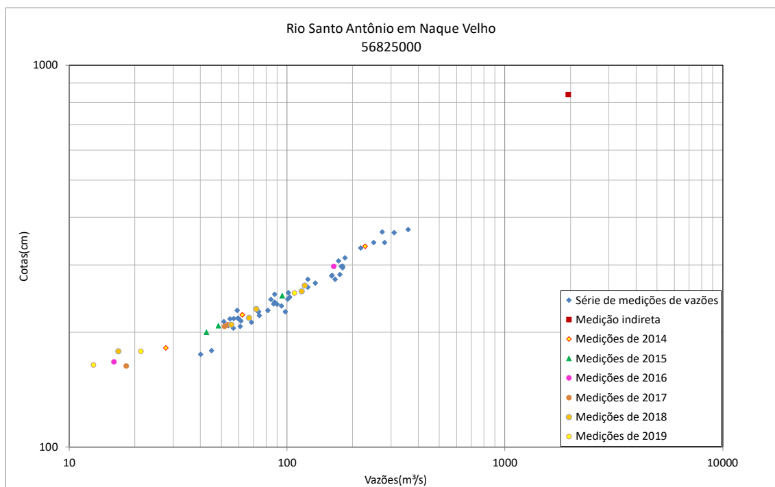
Figura 42 - Resumo de medições de descarga no Santo Antônio em Naque Velho (56825000)
