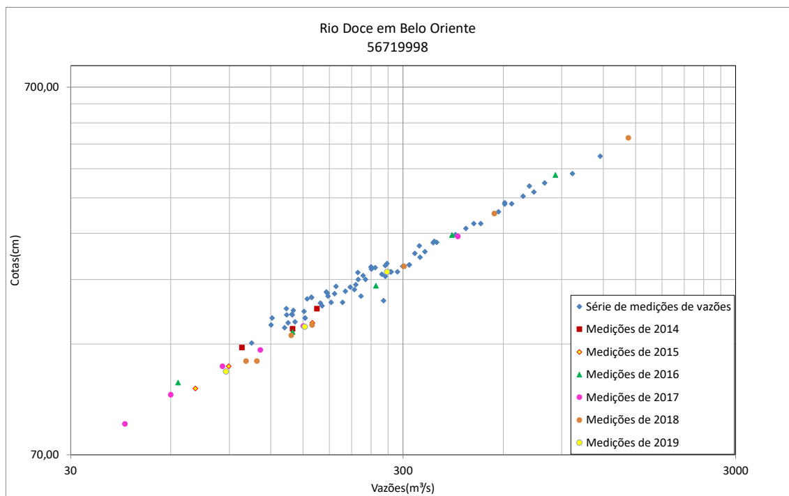
Figura 41 - Resumo de medições de descarga no rio Doce em Belo Oriente (56719998)
