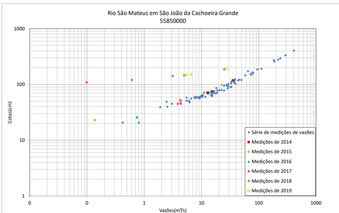
Figura 40 - Resumo de medições de descarga no rio São Mateus em São João da Cachoeira Grande
