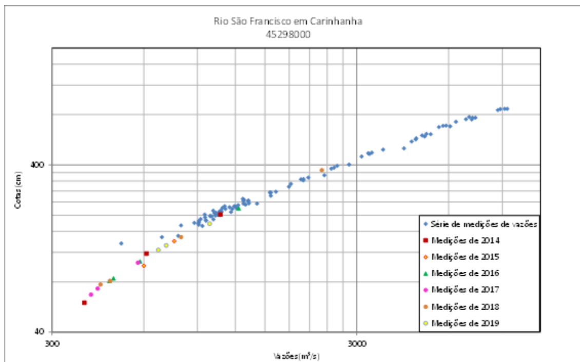
Figura 35 - Resumo de medições de descarga no rio São Francisco em Carinhanha (45298000)
