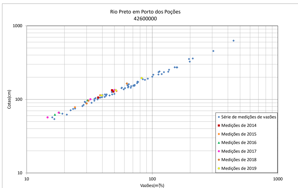
Figura 31 - Resumo de medições de descarga no rio Preto em Porto dos Poções (42600000)
