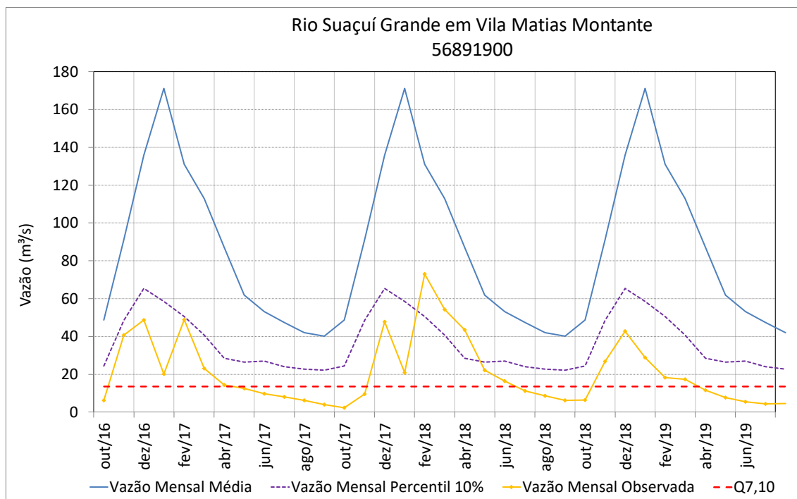
Figura 86 – Vazões médias mensais do rio Suaçuí Grande em Vila Matias Montante
