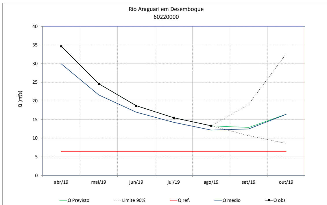
Figura 89 – Previsão de vazões do rio Araguari em Desemboque
