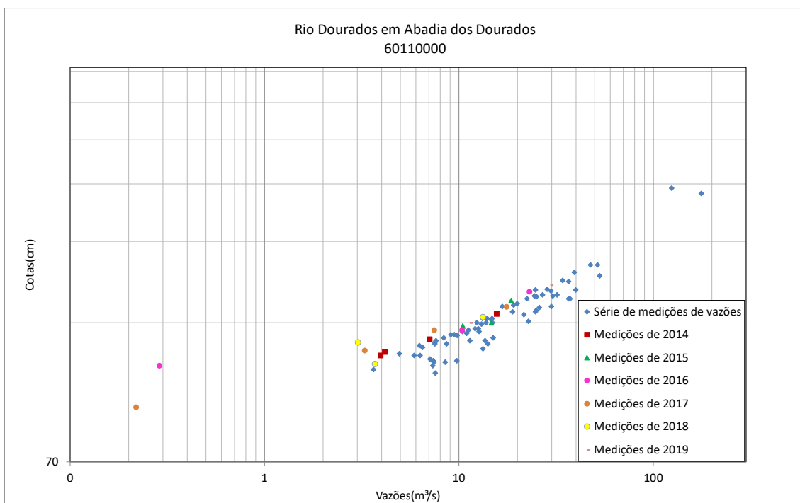
Figura 46 - Resumo de medições de descarga no rio Dourados em Abadia dos Dourados (60110000)
