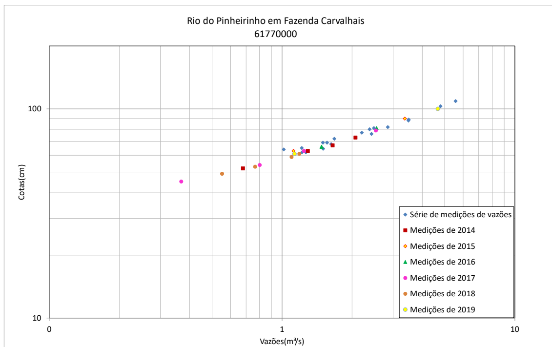
Figura 53 - Resumo de medições de descarga no rio Pinheirinho em Fazenda Carvalhais (61770000)
