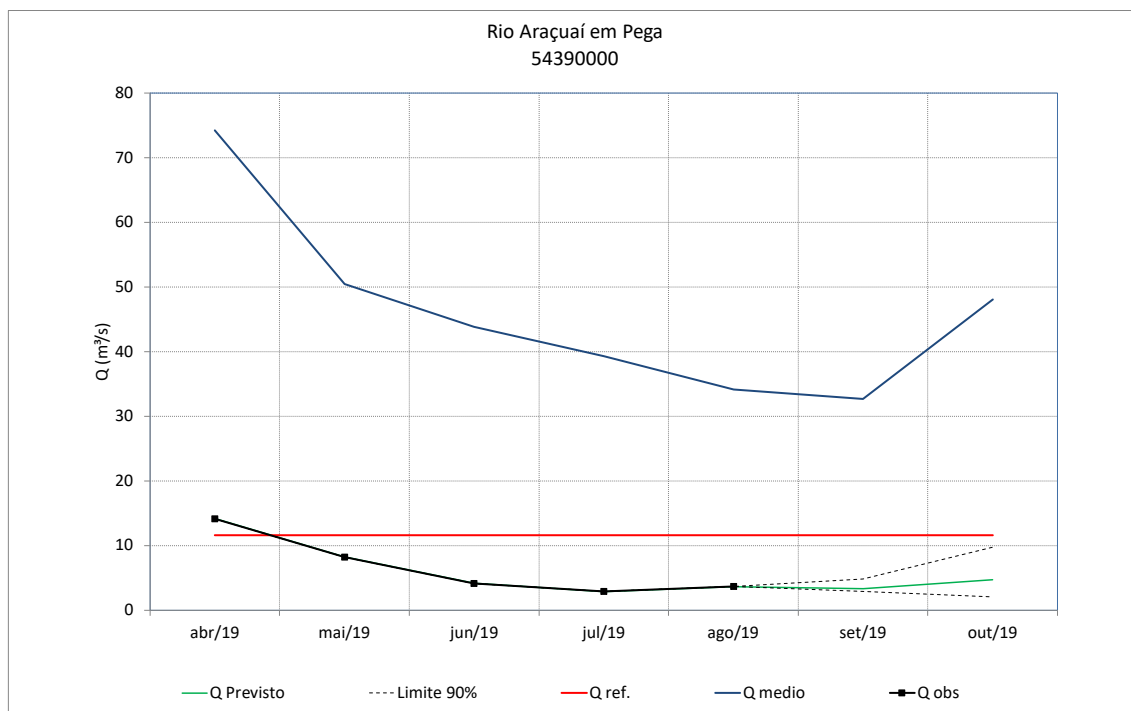
Figura 78 – Previsão de vazões do rio Araçuaí em Pega
