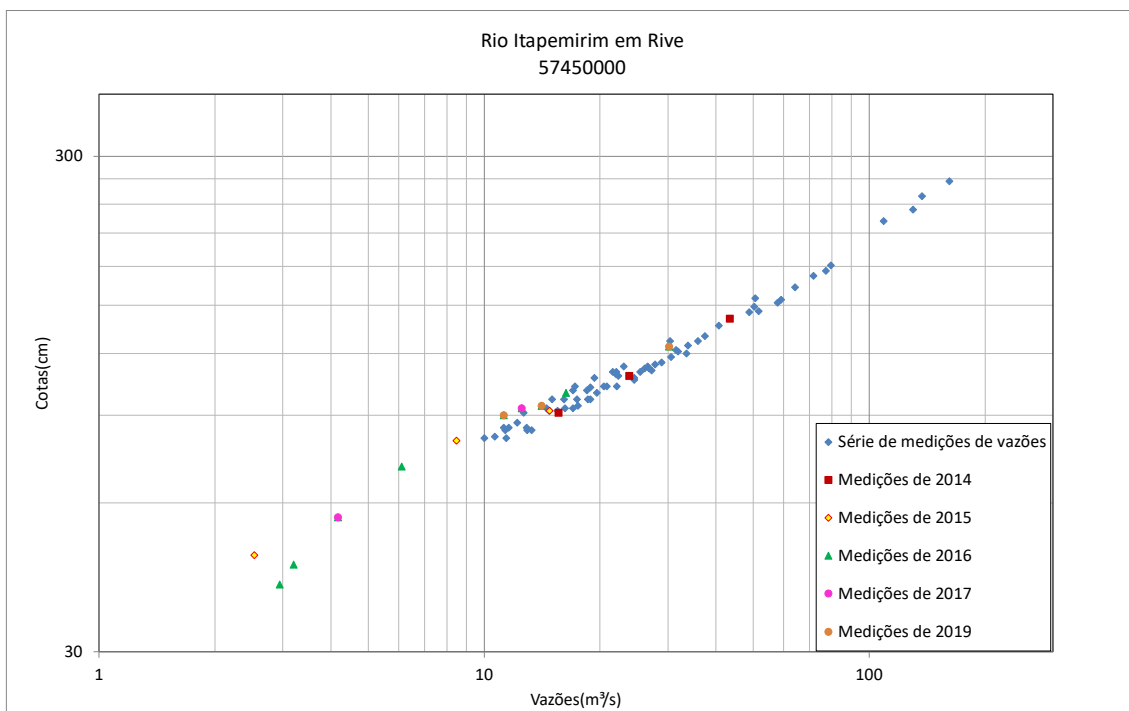
Figura 45 - Resumo de medições de descarga no rio Itapemirim em Rive (57450000)
