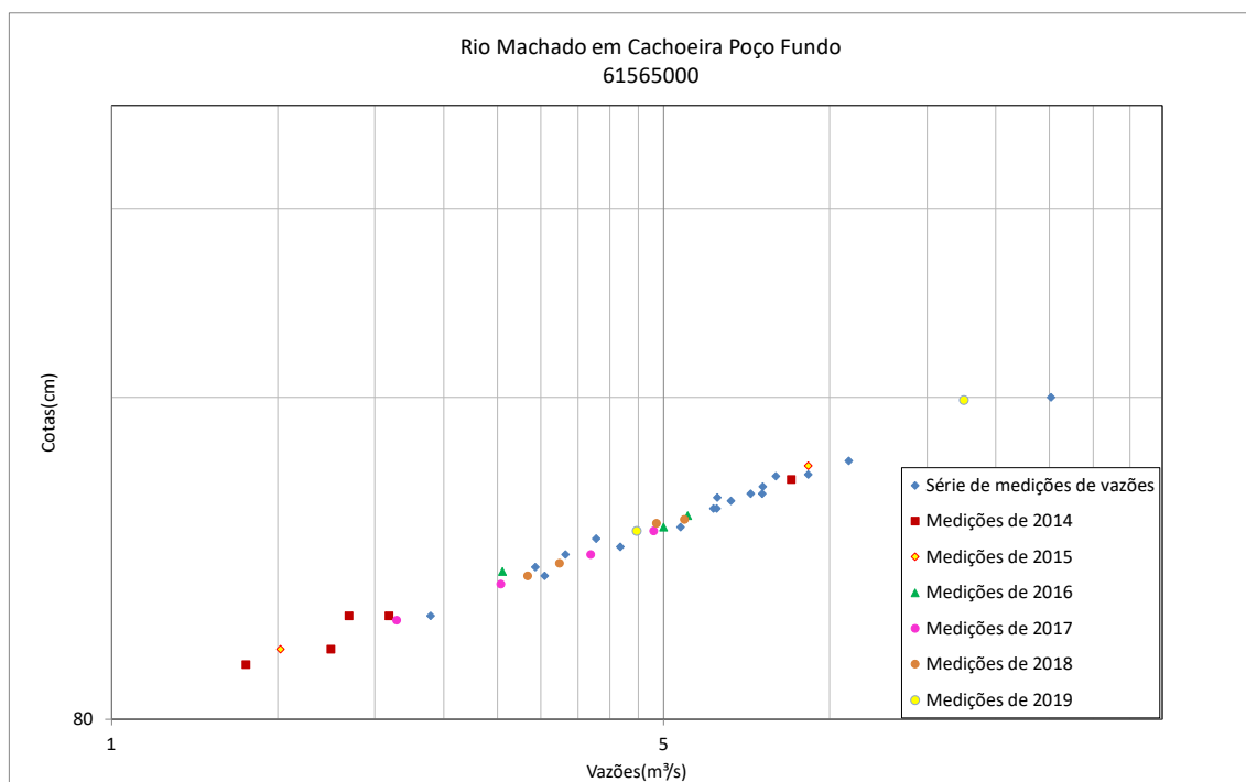
Figura 52 - Resumo de medições de descarga no rio Machado em Cachoeira Poço Fundo (61565000)
