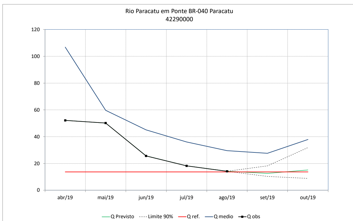
Figura 71 – Previsão de vazões do rio Paracatu em Ponte BR-040
