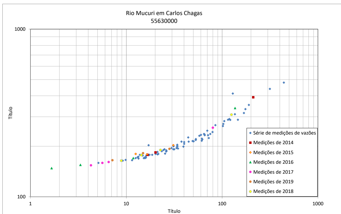
Figura 38 - Resumo de medições de descarga no rio Mucuri em Carlos Chagas (55630000)
