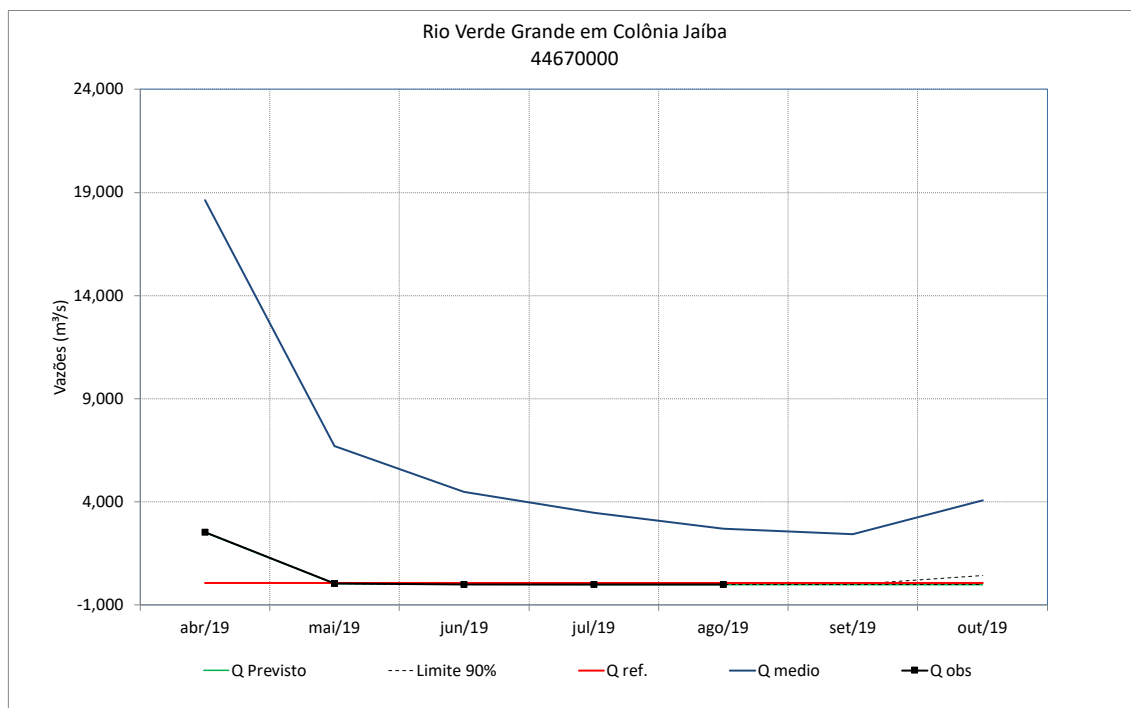
Figura 74 – Previsão de vazões do rio Verde Grande em Colônia do Jaíba
