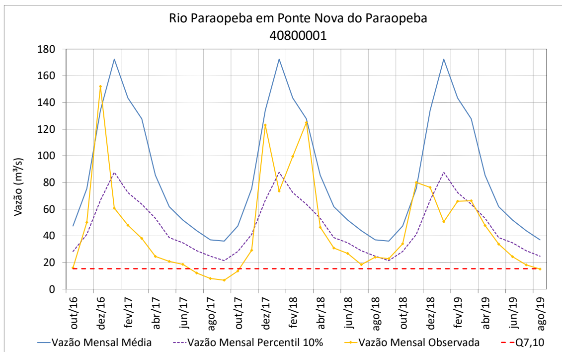
Figura 66 – Vazões médias mensais do rio Paraopeba em Ponte Nova do Paraopeba
