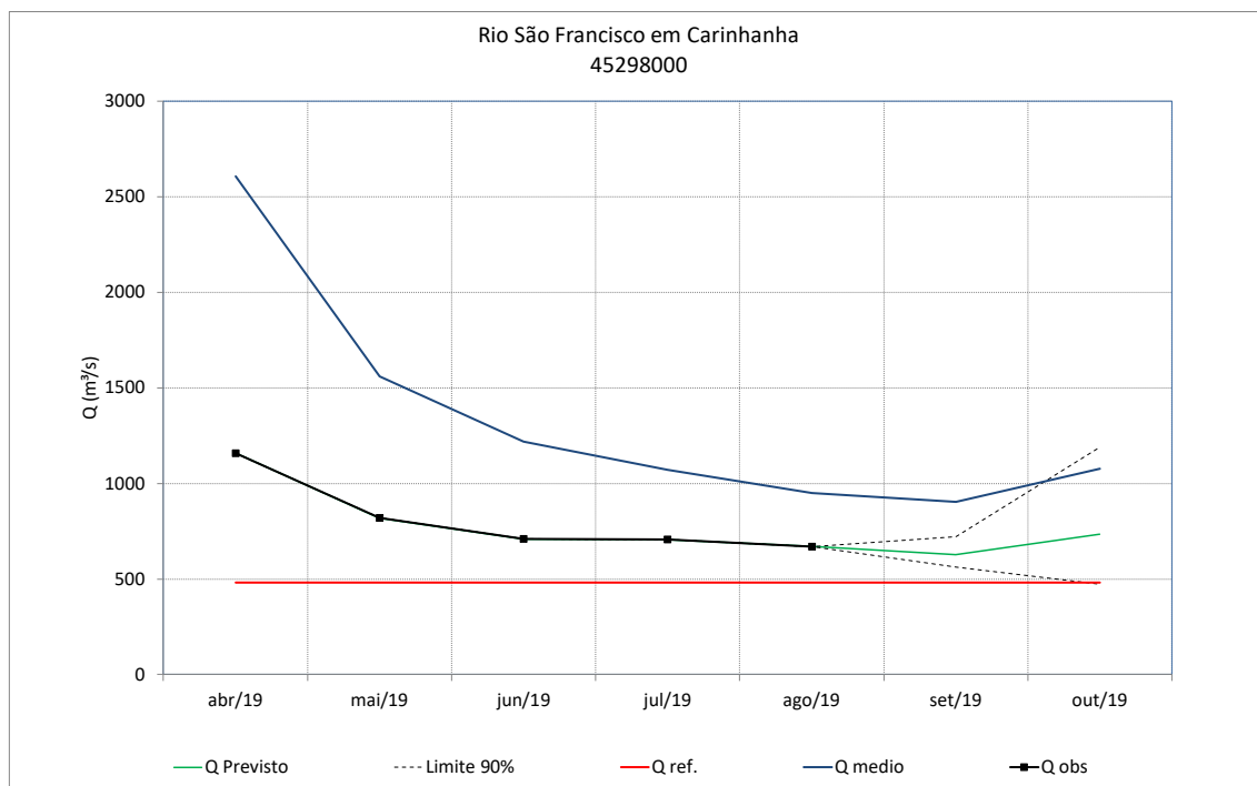
Figura 76 – Previsão de vazões do rio São Francisco em Carinhanha
