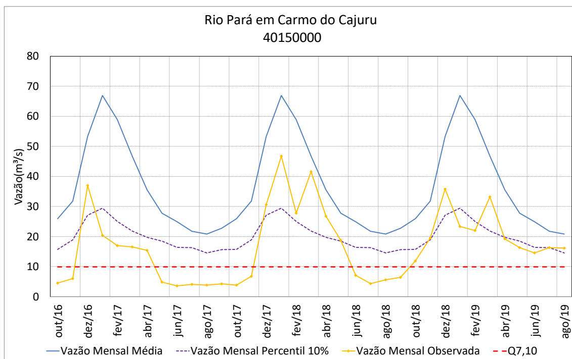
Figura 55 - Vazões médias mensais do rio Pará em Carmo do Cajuru
