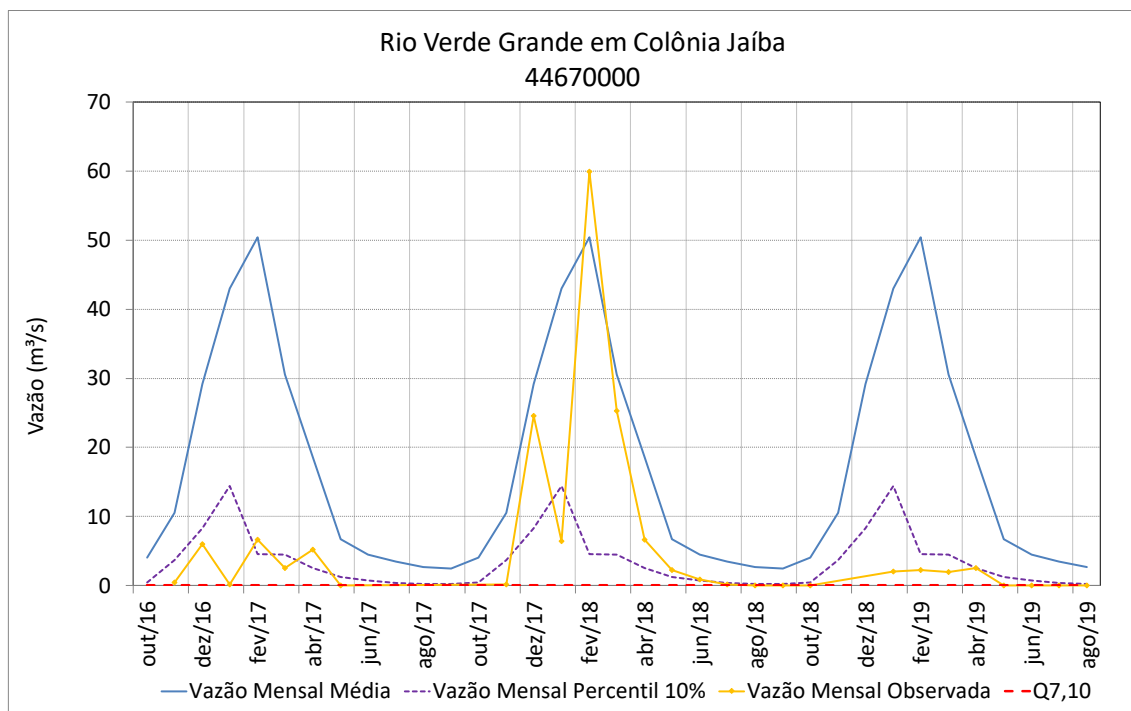
Figura 74 – Vazões médias mensais do rio Verde Grande em Colônia do Jaíba
