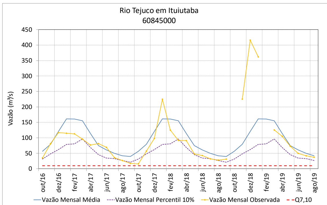
Figura 92 – Vazões médias mensais do rio Tejuco em Ituiutaba
