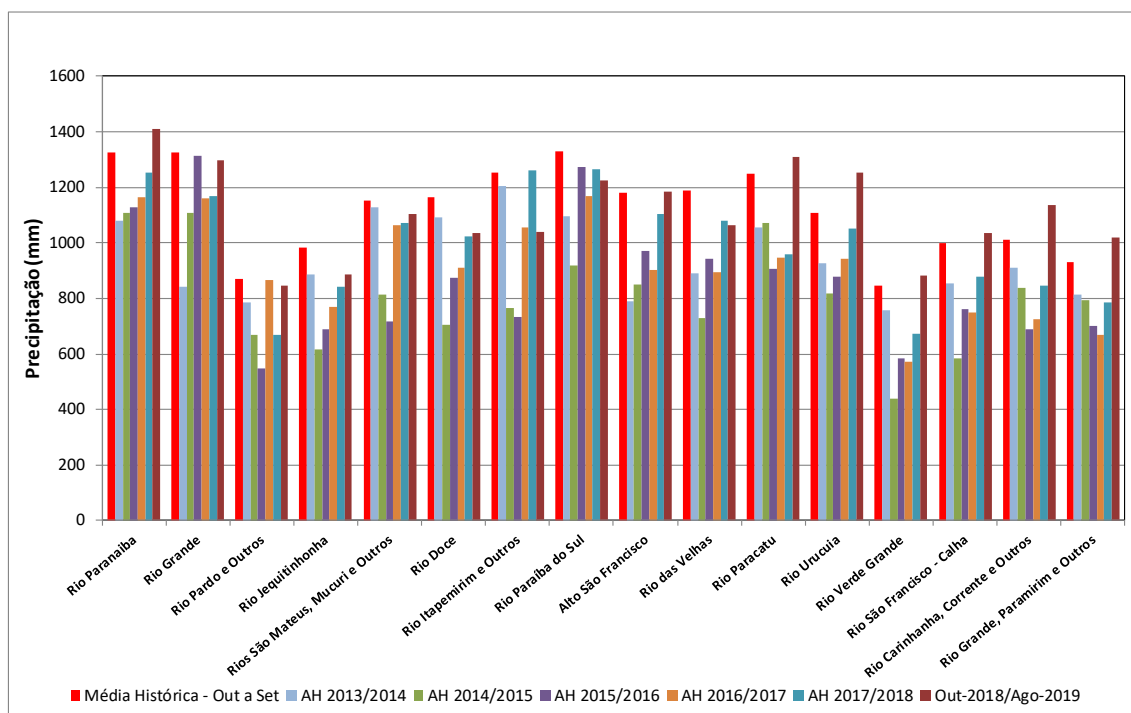
Figura 14 - Comparação entre a precipitação média acumulada nos anos hidrológicos 2013/2014, 2014/2015, 2015/2016 e 2016/2017, 2017/2018 e 2018/2019 (sem setembro).
