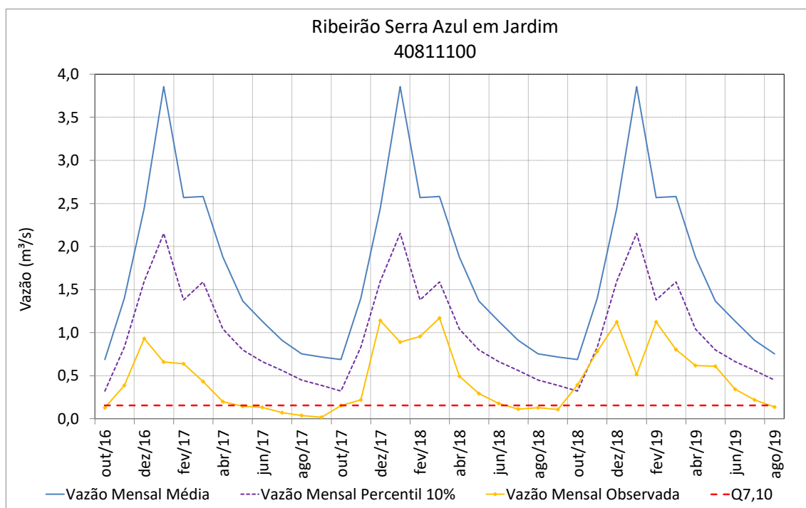
Figura 67 – Vazões médias do ribeirão Serra Azul em Jardim
