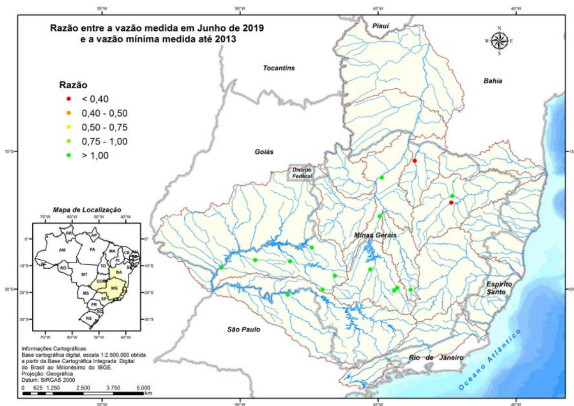
Figura 19 - Razão entre a vazão medida em junho de 2019 e a vazão mínima medida até 2013.
