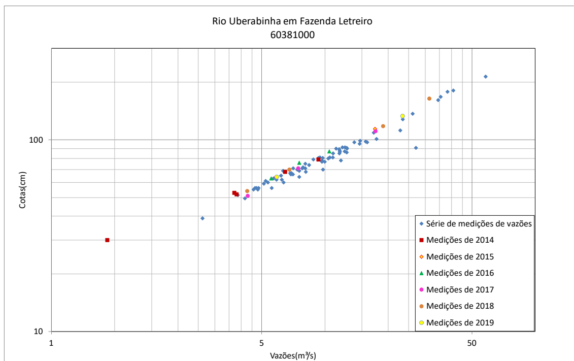
Figura 48 - Resumo de medições de descarga no rio Uberabinha em Fazenda Letreiro (60381000)
