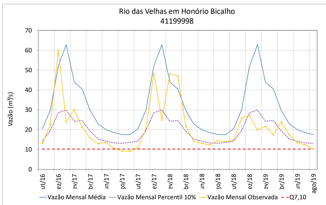
Figura 69 – Vazões médias mensais do rio das Velhas em Honório Bicalho
