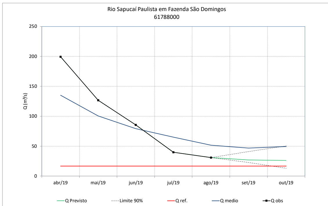
Figura 97 – Previsão de vazões do rio Sapucaí Paulista em Fazenda São Domingos
