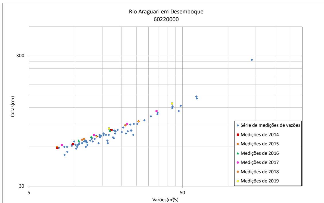
Figura 47 - Resumo de medições de descarga no rio Araguari em Desemboque (60220000)
