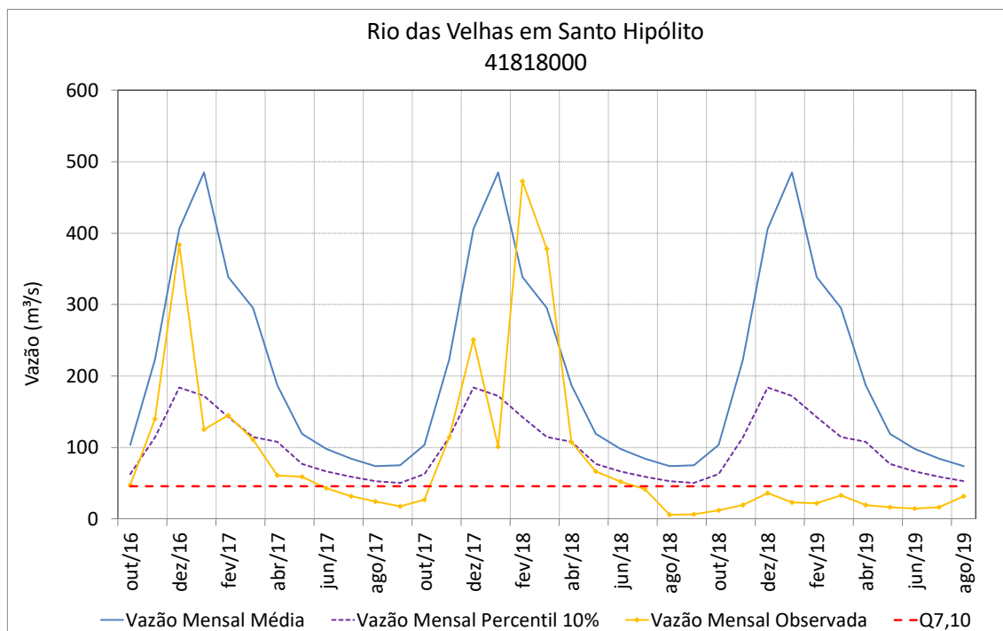
Figura 70 – Vazões médias mensais do rio das Velhas em Santo Hipólito
