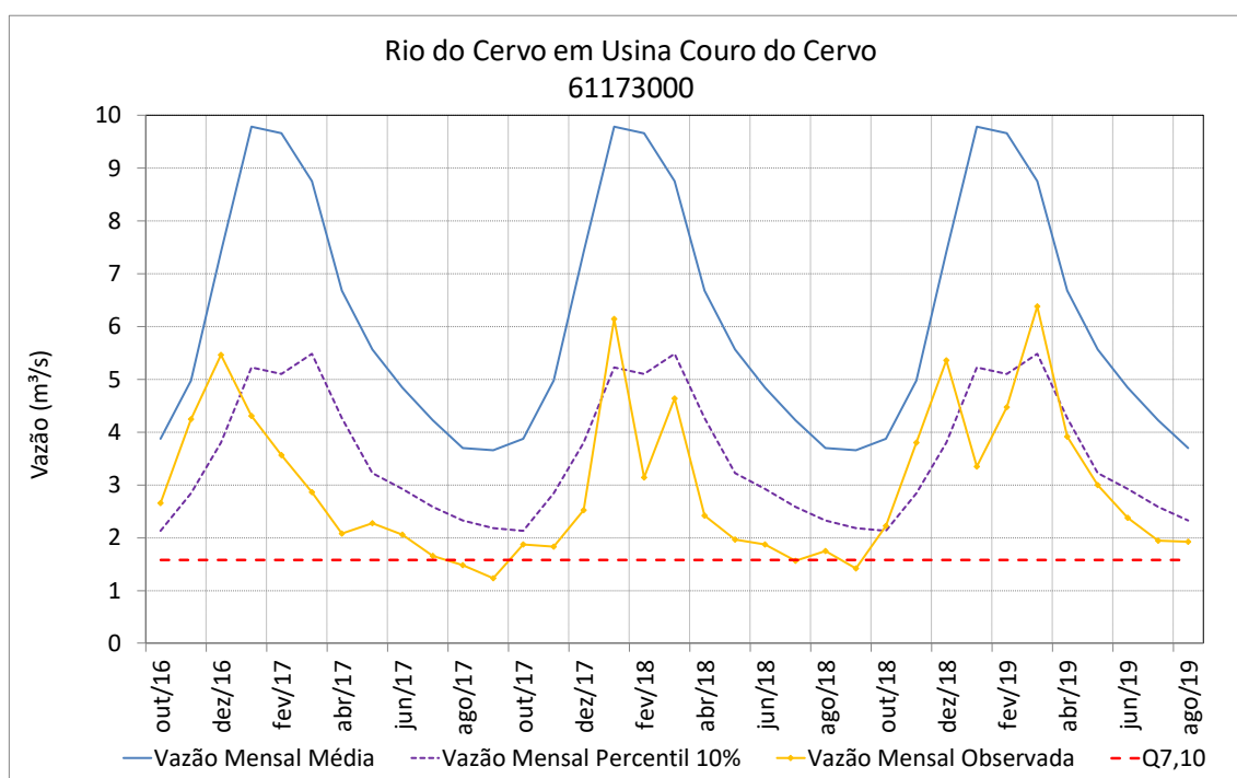
Figura 94 – Vazões médias mensais do rio do Cervo em Usina Couro do Cervo
