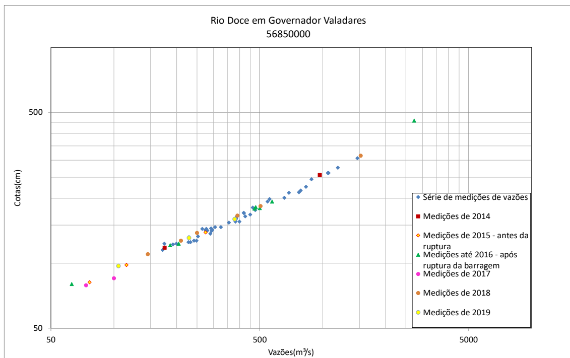
Figura 43 - Resumo de medições de descarga no Doce em Governador Valadares (56850000)
