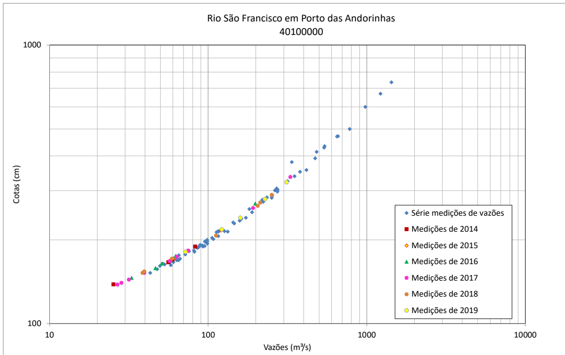
Figura 22 - Resumo de medições de descarga no rio São Francisco em Porto das Andorinhas (40100000)
