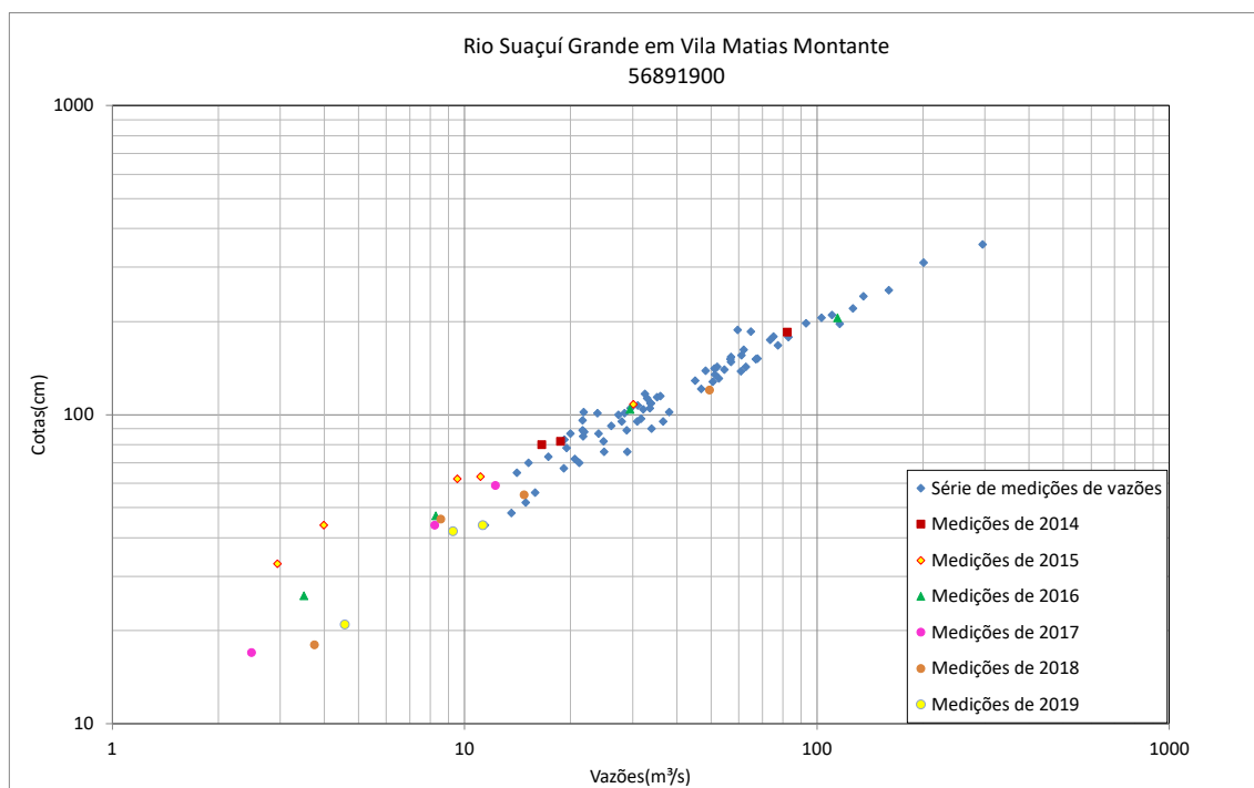
Figura 44 - Resumo de medições de descarga no Suaçuí Grande em Vila Matias Montante (56891900)
