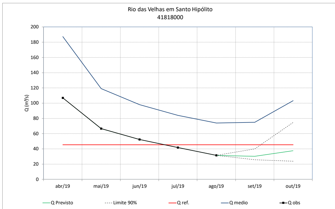
Figura 70 – Previsão de vazões do rio das Velhas em Santo Hipólito
