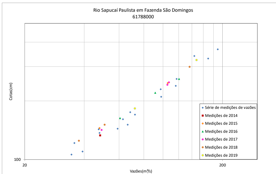
Figura 54 - Resumo de medições de descarga no rio Sapucaí em Fazenda São Domingos (61788000)
