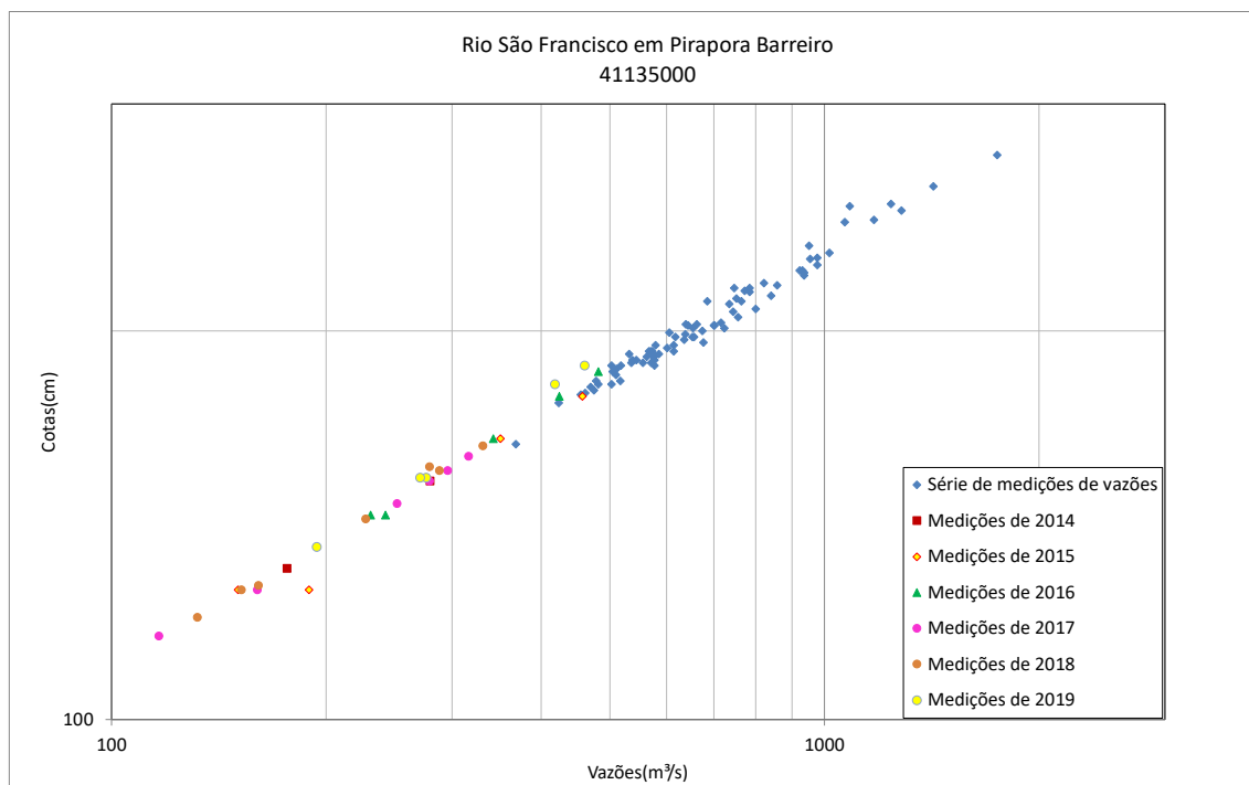
Figura 26 - Resumo de medições de descarga no rio São Francisco em Pirapora Barreiro (41135000)
