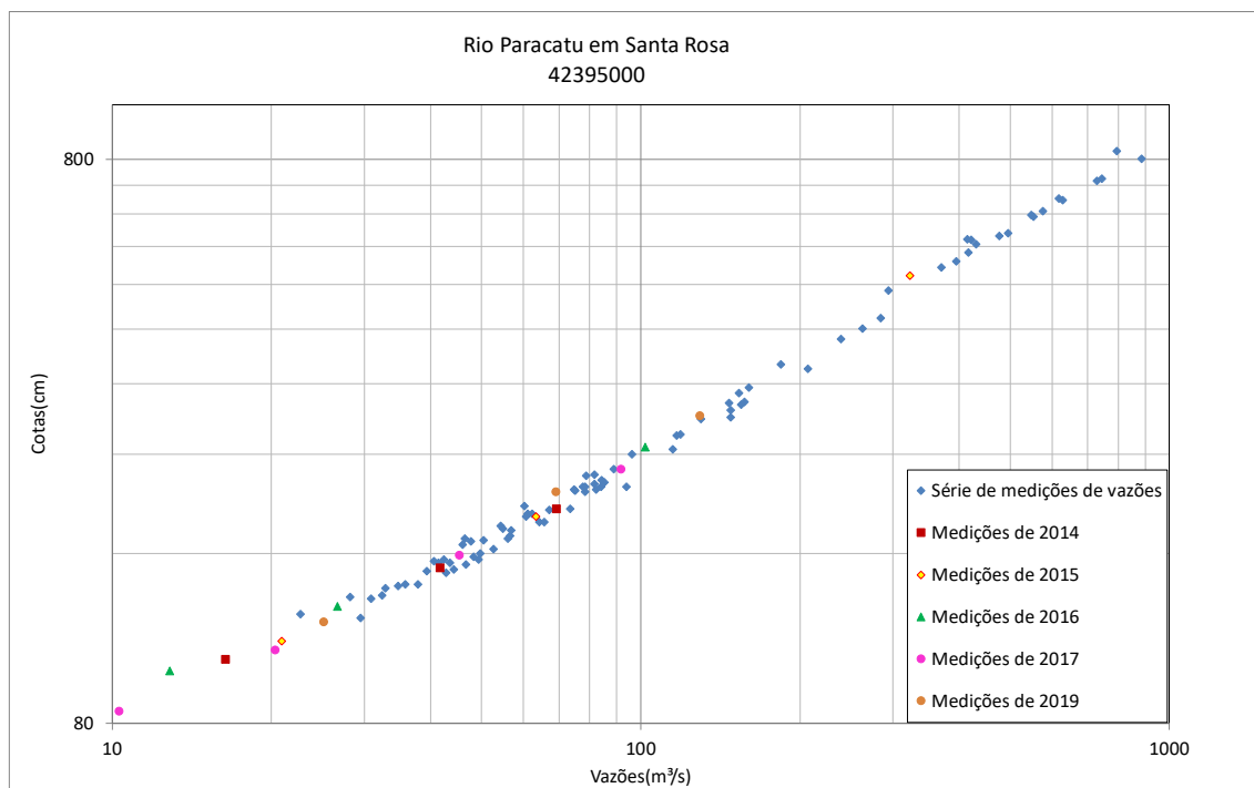
Figura 30 - Resumo de medições de descarga no rio Paracatu em Santa Rosa (42395000)
