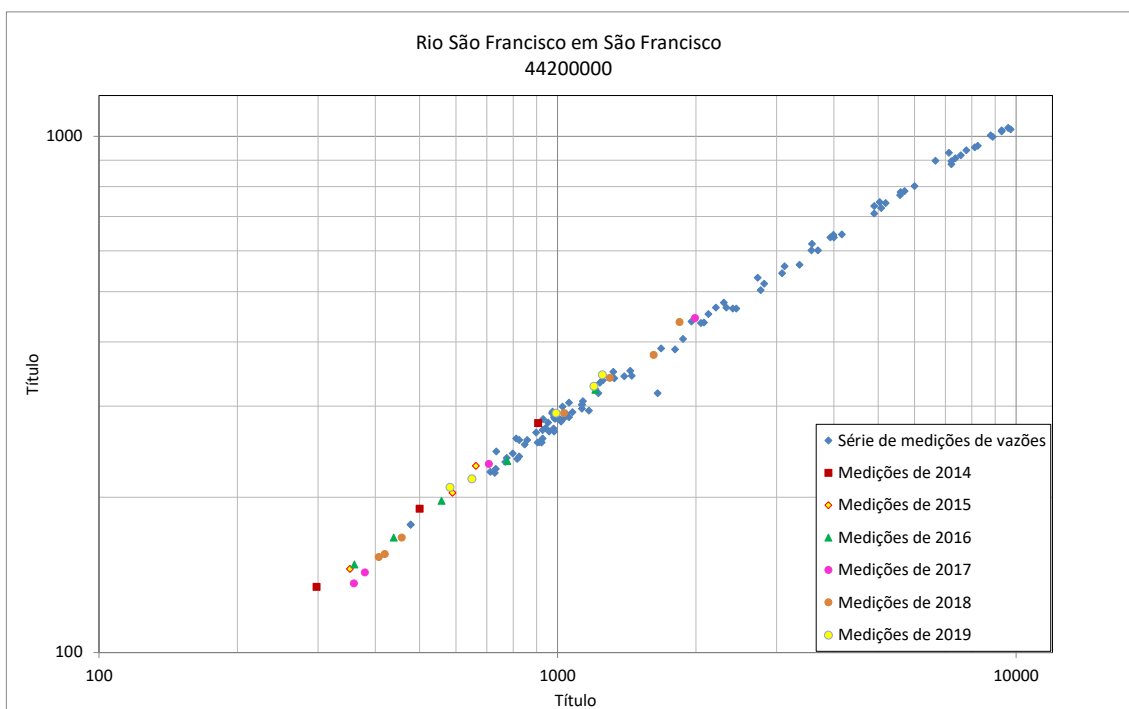
Figura 33 - Resumo de medições de descarga no rio São Francisco em São Francisco (44200000)
