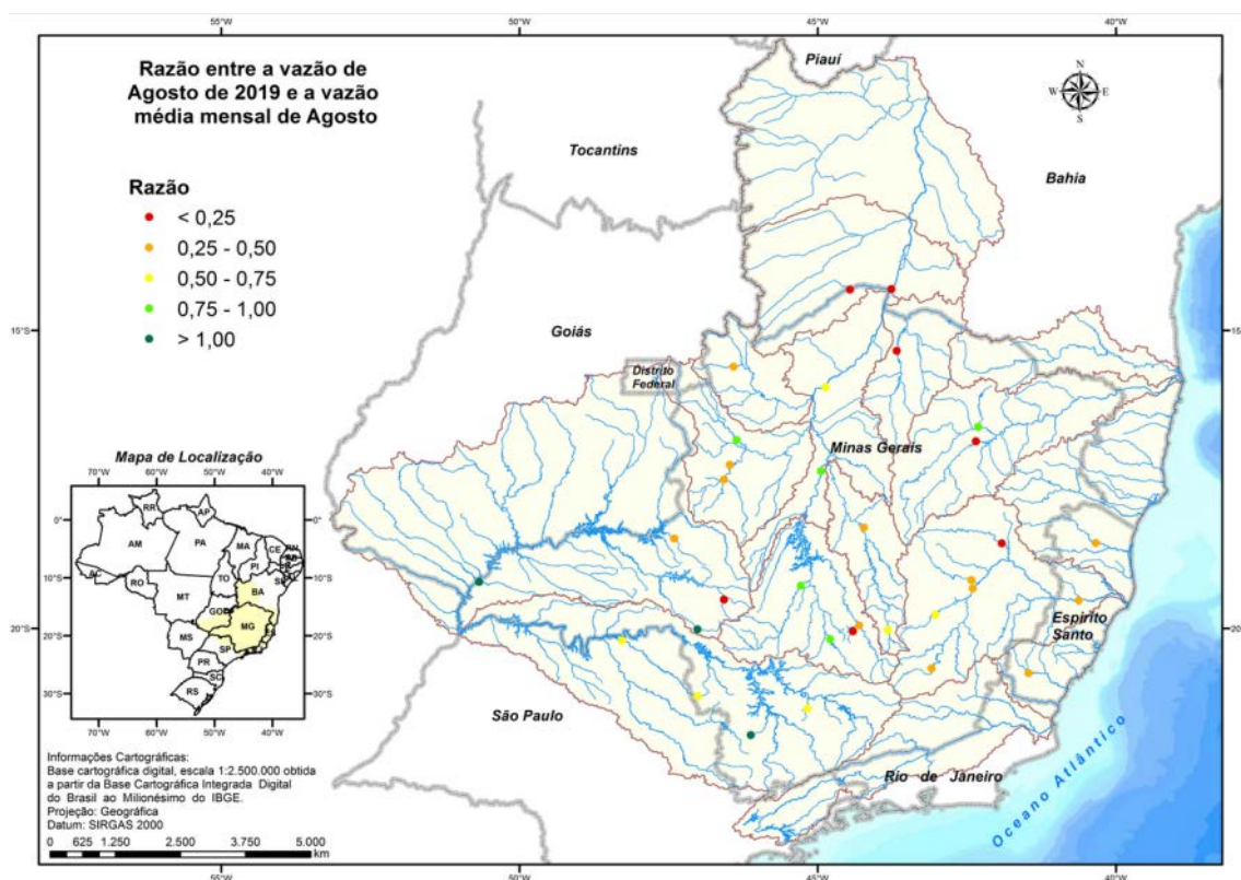
Figura 16 - Razão entre a vazão de agosto de 2019 e a vazão média mensal de agosto.
