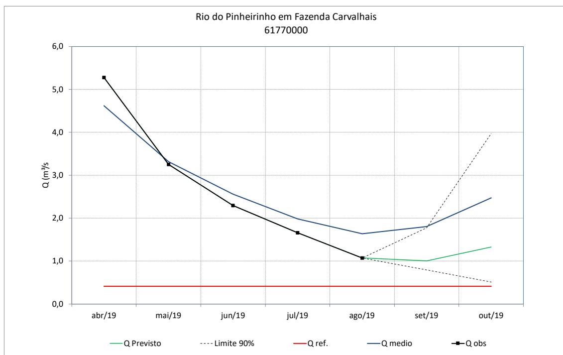
Figura 96 – Previsão de vazões do rio do Pinheirinho em Fazenda Carvalhais
