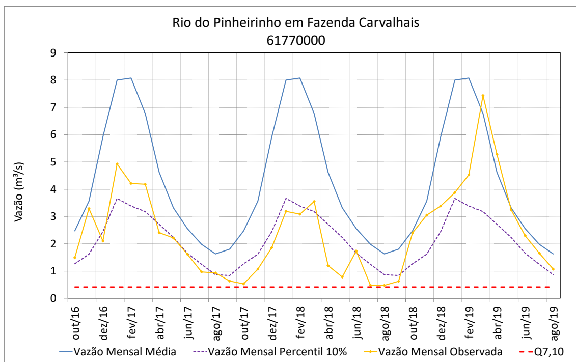
Figura 96 – Vazões médias mensais do rio do Pinheirinho em Fazenda Carvalhais
