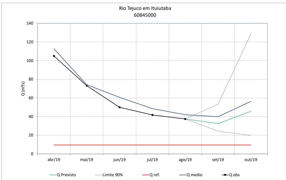
Figura 92 – Previsão de vazões do rio Tejuco em Ituiutaba
