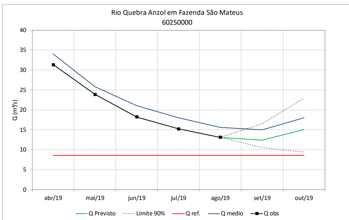
Figura 90 – Previsão de vazões do rio Quebra Anzol em Fazenda São Mateus
