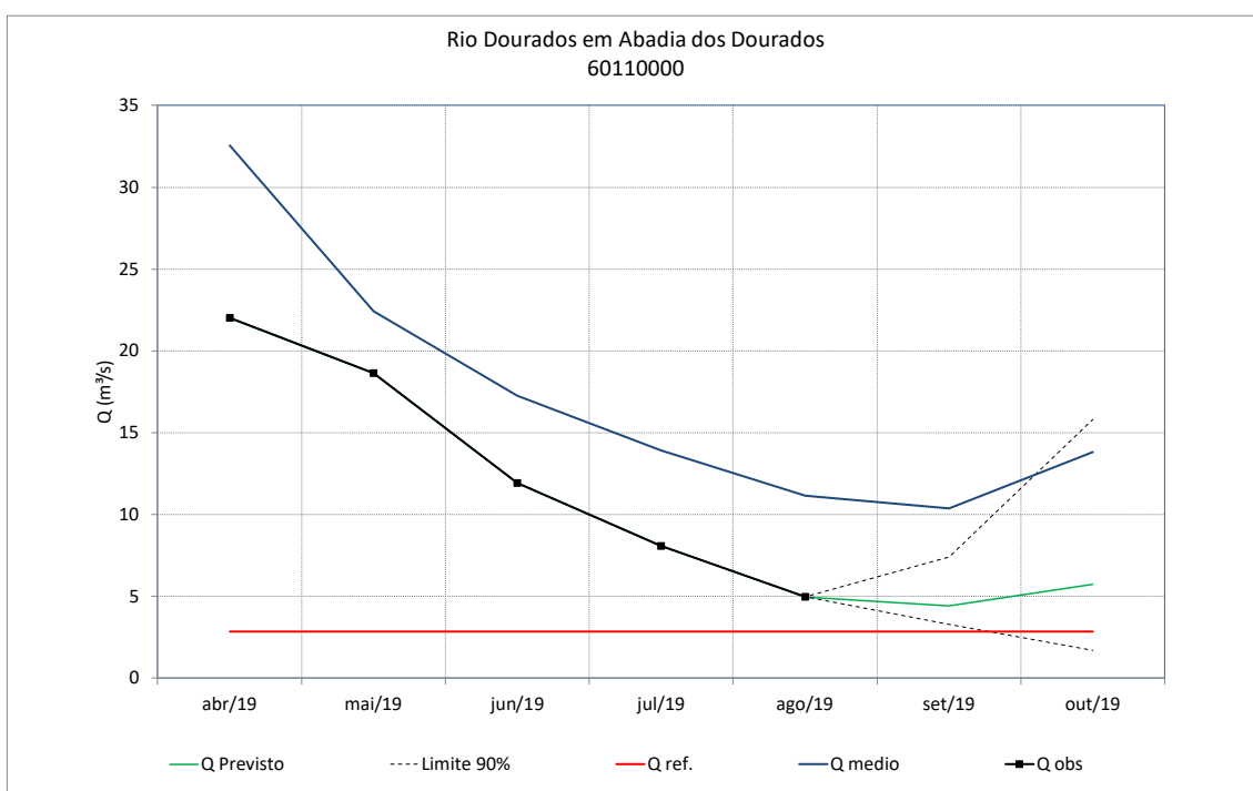
Figura 88 – Previsão de vazões do rio Dourados em Abadia dos Dourados
