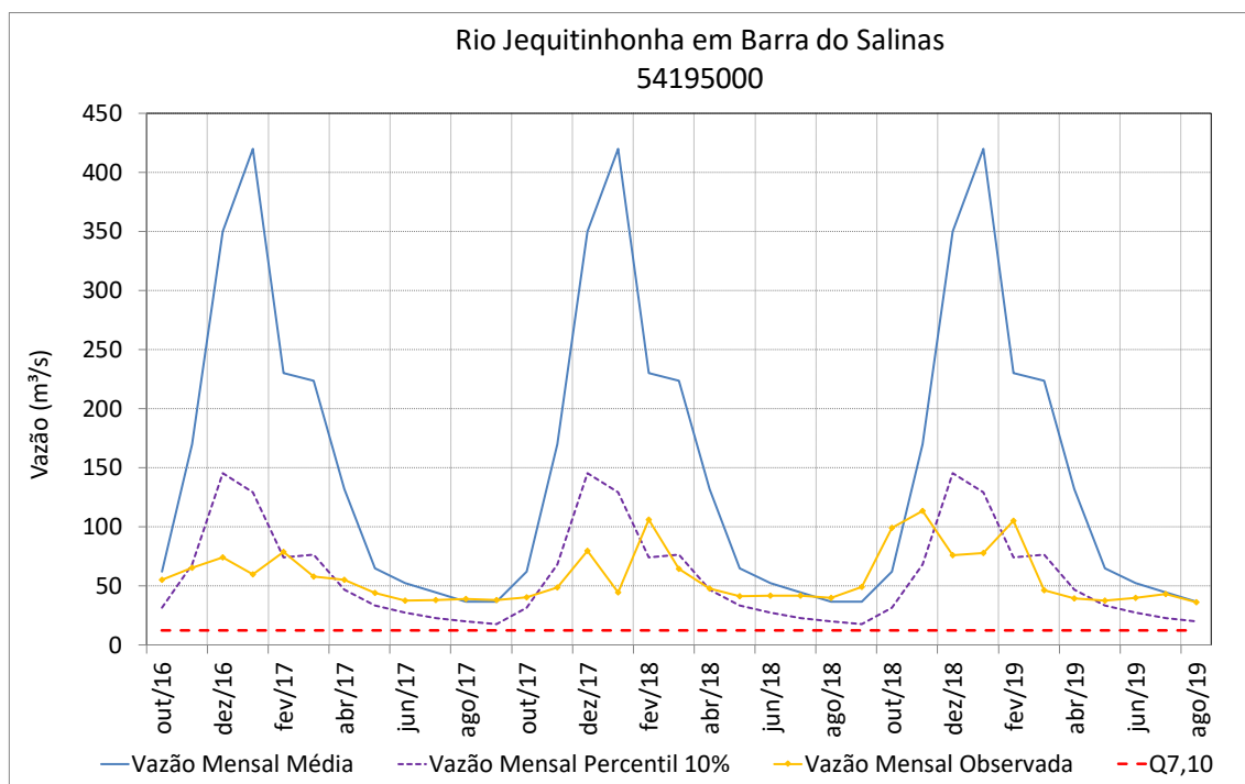
Figura 77 – Vazões médias mensais do rio Jequitinhonha em Barra do Salinas
