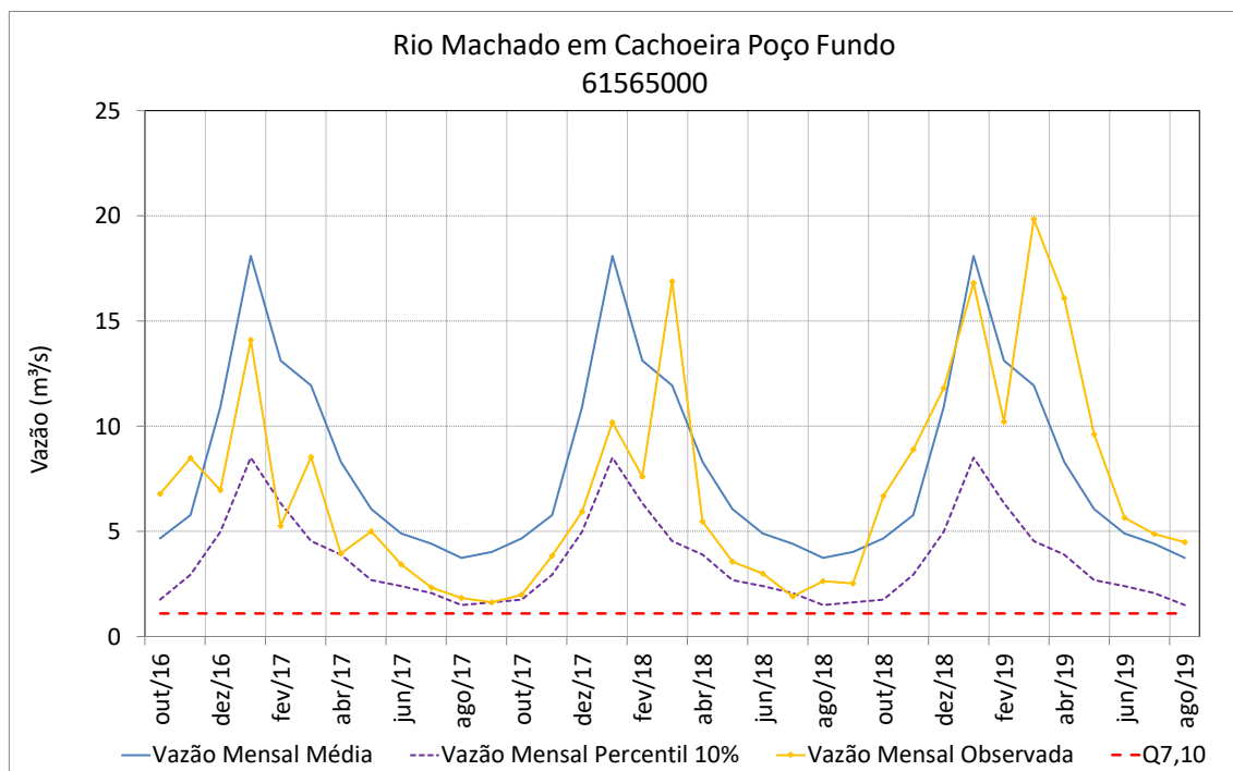
Figura 95 – Vazões médias mensais do rio Machado em Cachoeira Poço Fundo
