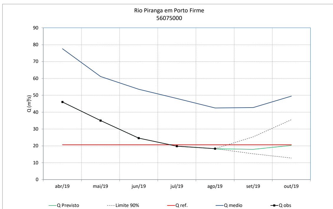
Figura 81 – Previsão de vazões do rio Piranga em Porto Firme
