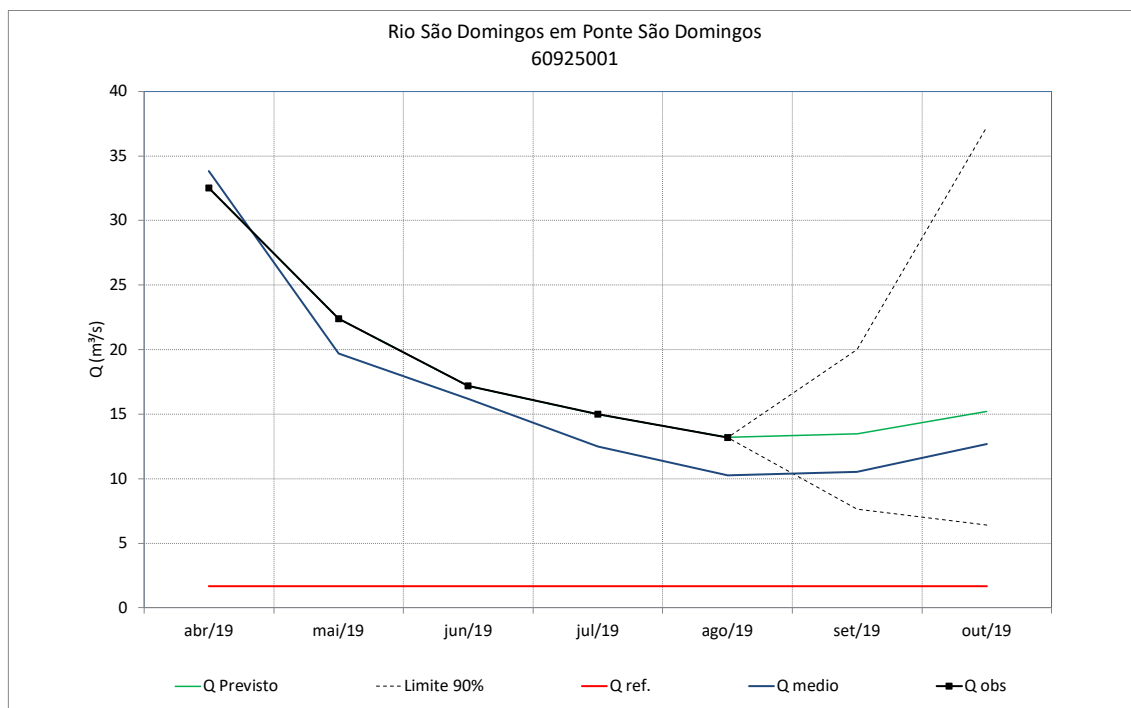
Figura 93 – Previsão de vazões do rio São Domingos em Ponte São Domingos
