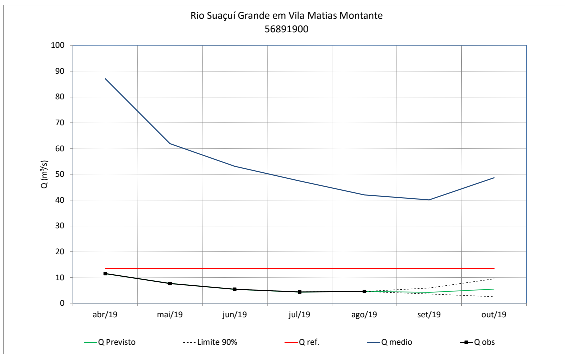
Figura 86 – Previsão de vazões do rio Suaçuí Grande em Vila Matias Montante
