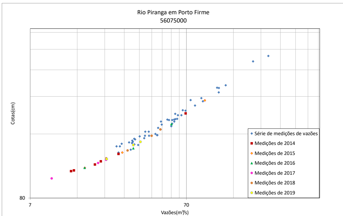
Figura 39 - Resumo de medições de descarga no rio Piranga em Porto Firme (56075000)
