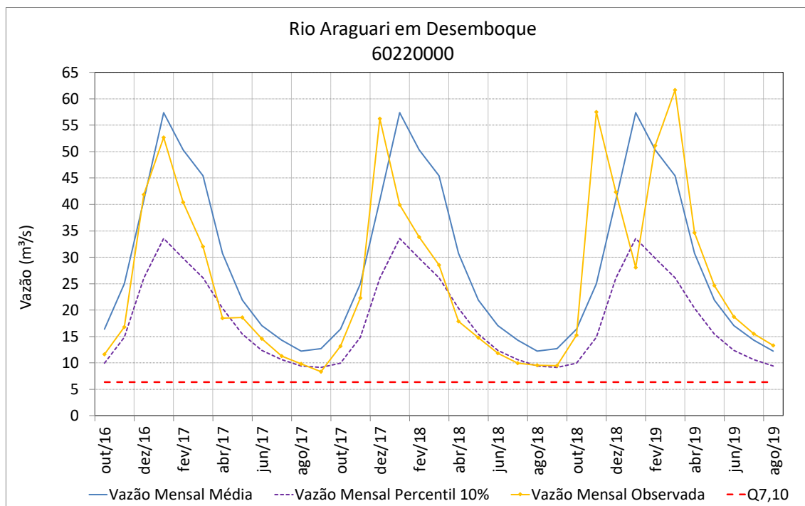
Figura 89 – Vazões médias mensais do rio Araguari em Desemboque
