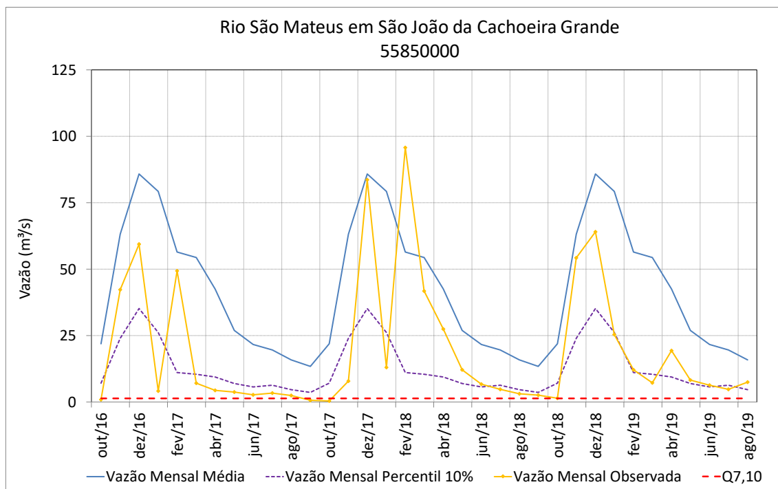
Figura 80 – Vazões médias mensais do rio São Mateus em São João da Cachoeira Grande
