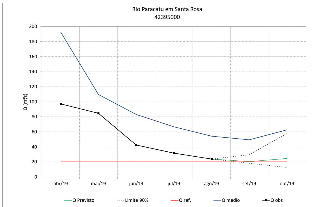
Figura 71 – Previsão de vazões do rio Paracatu em Santa Rosa
