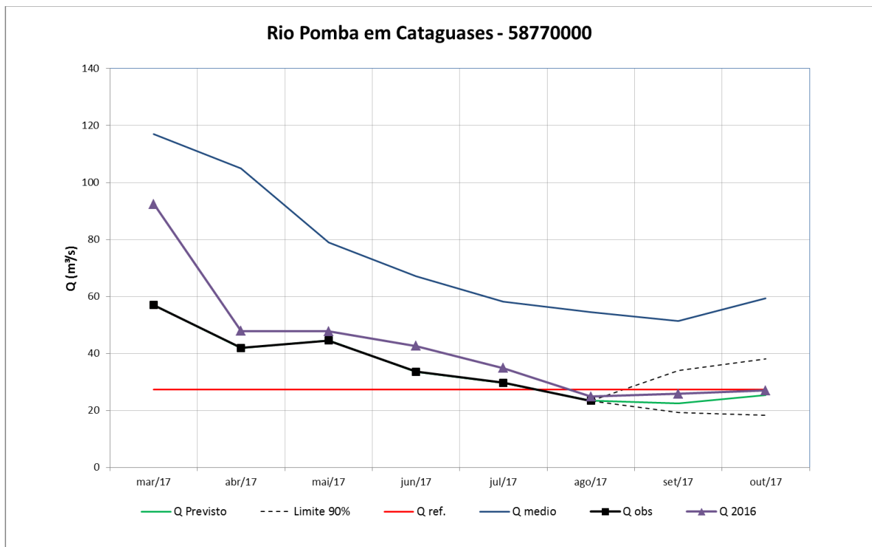
Figura 27 – Prognóstico de vazão para a estação de Cataguases
