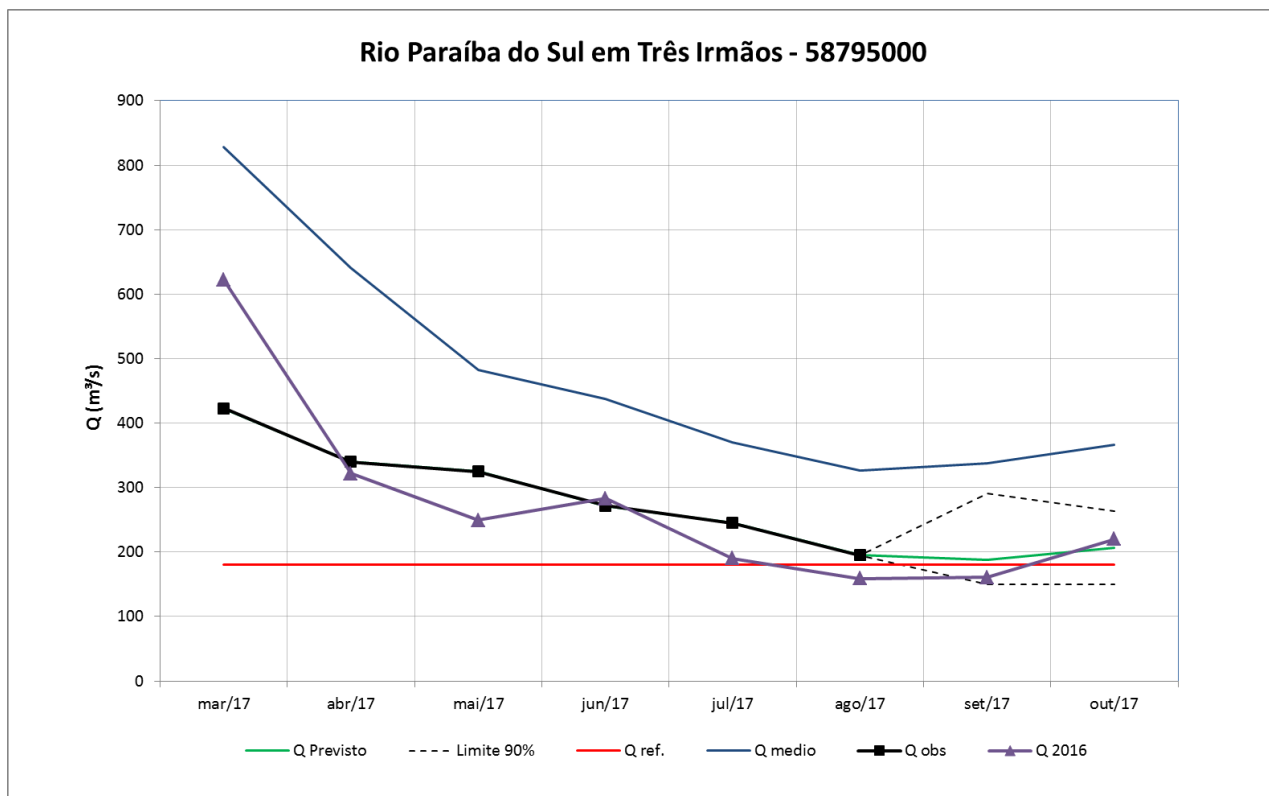
Figura 30 – Prognóstico de vazão para a estação de Três Irmãos
