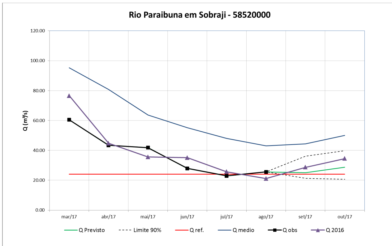
Figura 33 – Prognóstico de vazão para a estação de Sobraji
