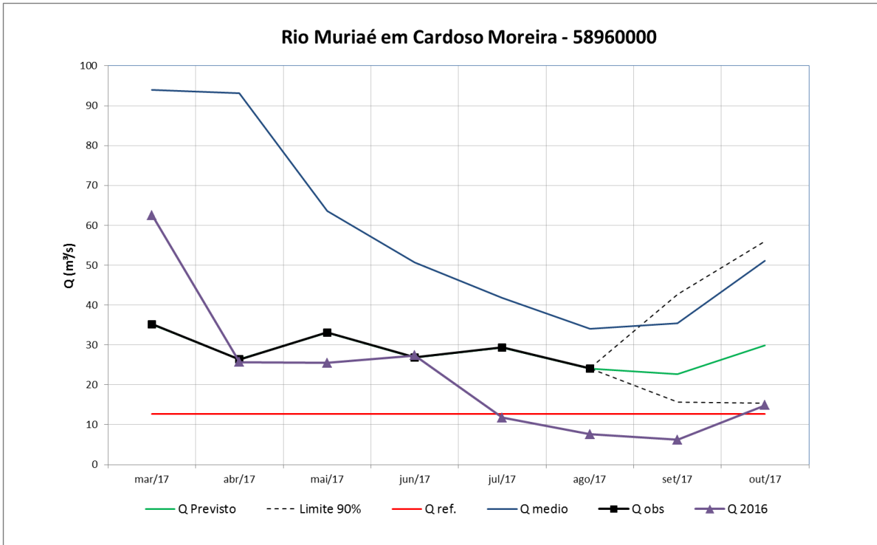
Figura 28 – Prognóstico de vazão para a estação de Cardoso Moreira
