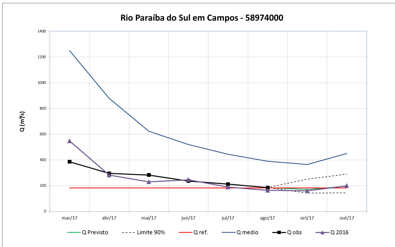
Figura 31 – Prognóstico de vazão para a estação de Campos
