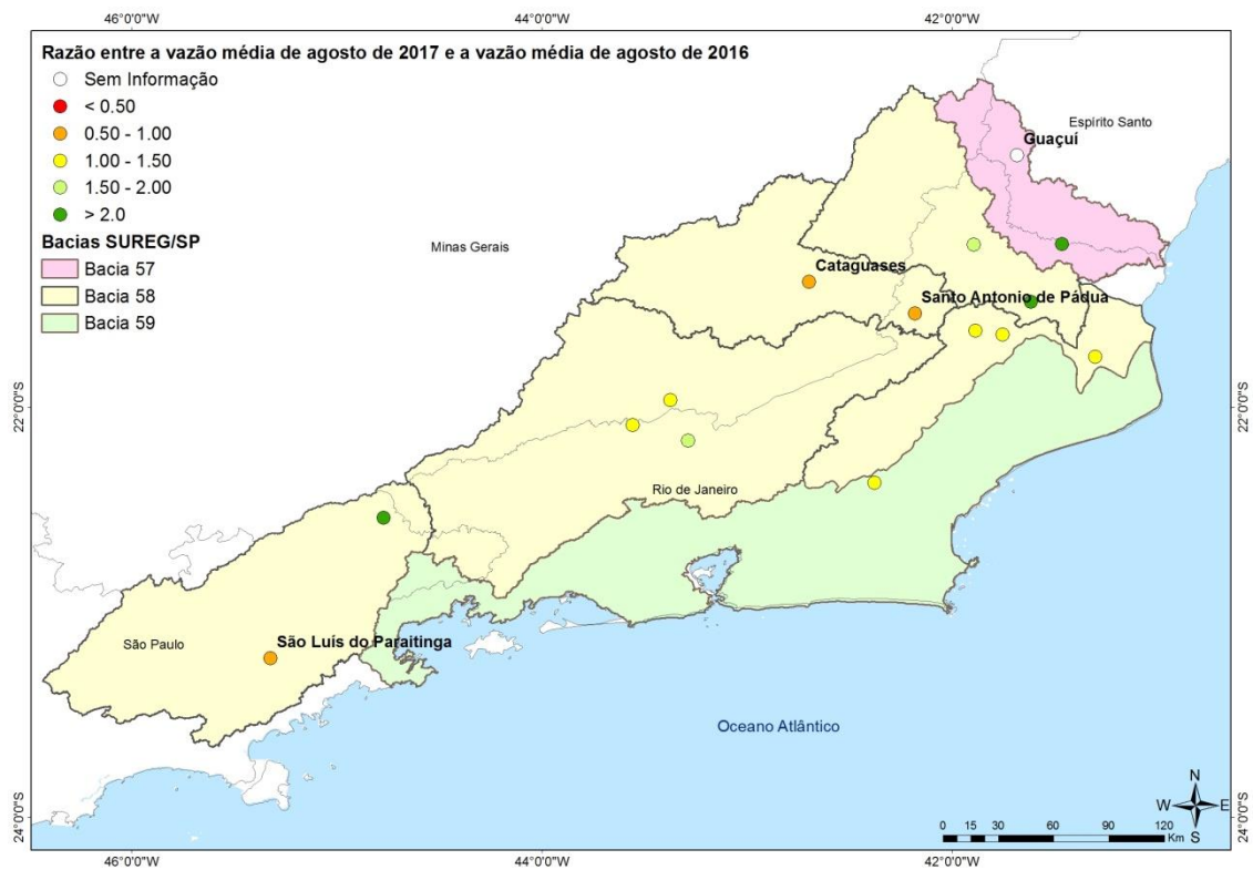
Figura 10 – Comparação entre a vazão de agosto de 2017 e a vazão de agosto de 2016
