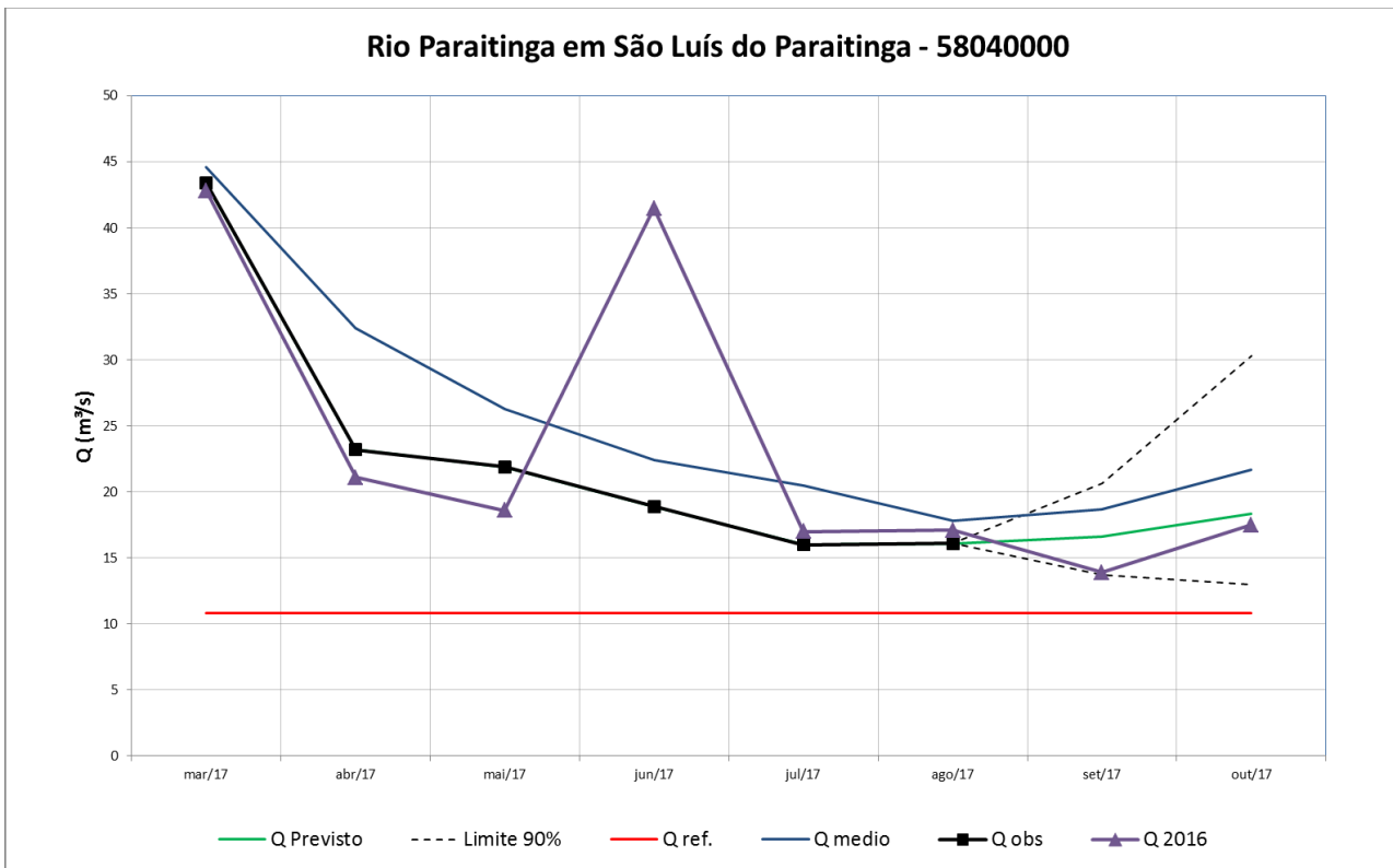
Figura 37 – Prognóstico de vazão para a estação de São Luís do Paraitinga
