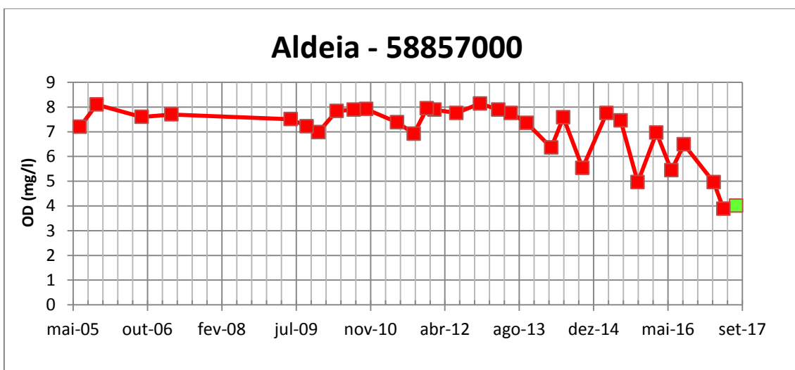
Figura 18 - Série histórica de OD na estação Aldeia
