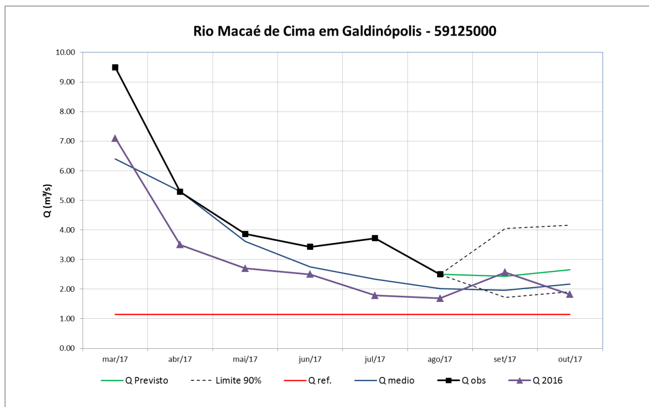
Figura 38 – Prognóstico de vazão para a estação de Galdinópolis
