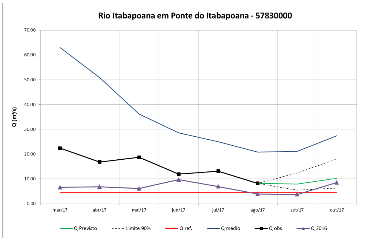
Figura 26 – Prognóstico de vazão para a estação de Ponte do Itabapoana
