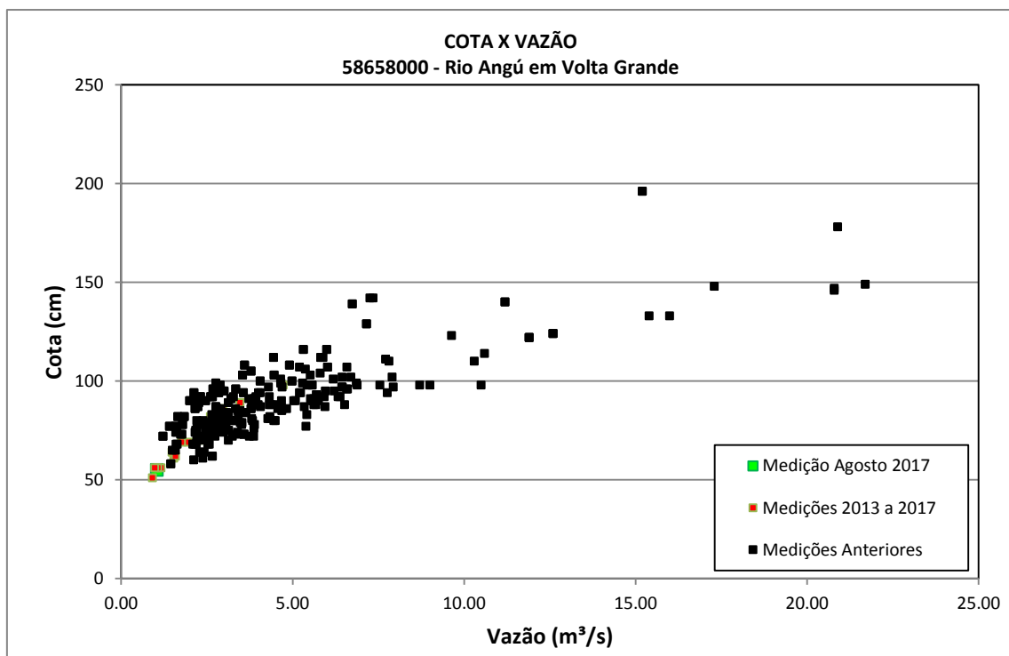
Figura 13 – Gráfico Cota x Vazão na estação Volta Grande
