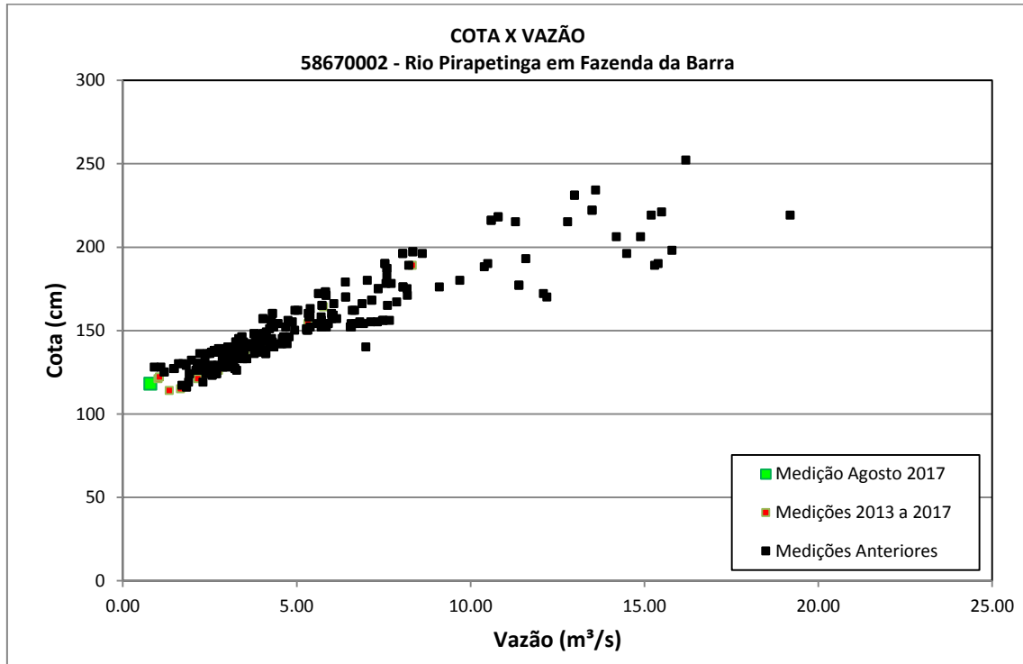
Figura 12 – Gráfico Cota x Vazão na estação Fazenda da Barra
