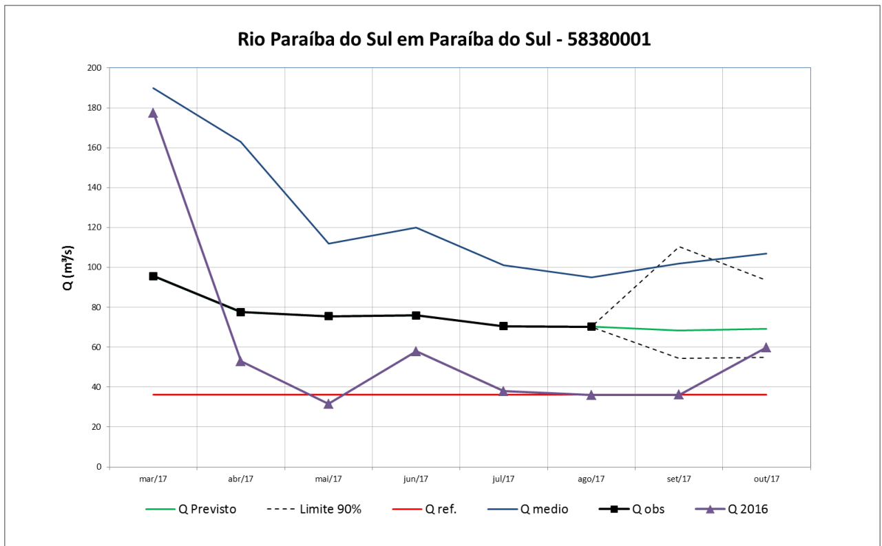
Figura 35 – Prognóstico de vazão para a estação de Paraíba do Sul
