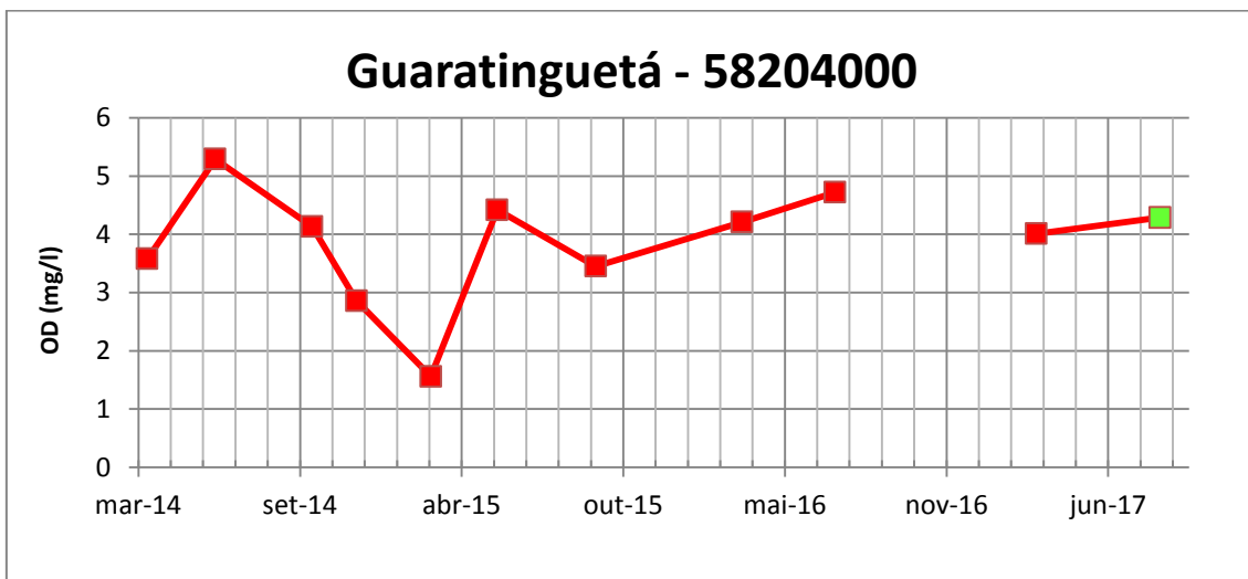
Figura 20 - Série histórica de OD na estação Guaratinguetá
