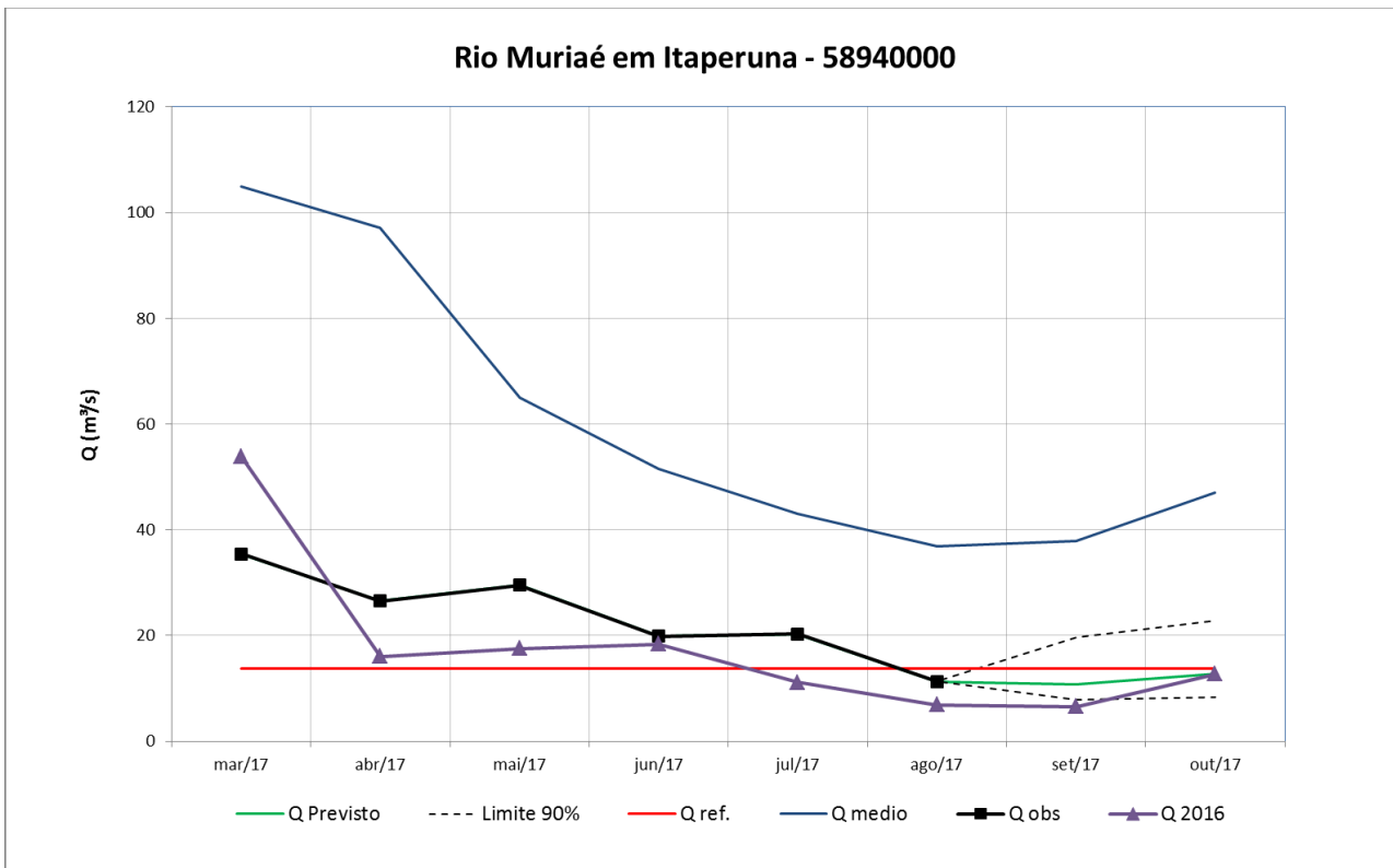
Figura 29 – Prognóstico de vazão para a estação de Itaperuna
