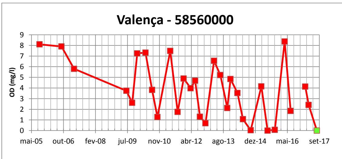
Figura 19 - Série histórica de OD na estação Valença
