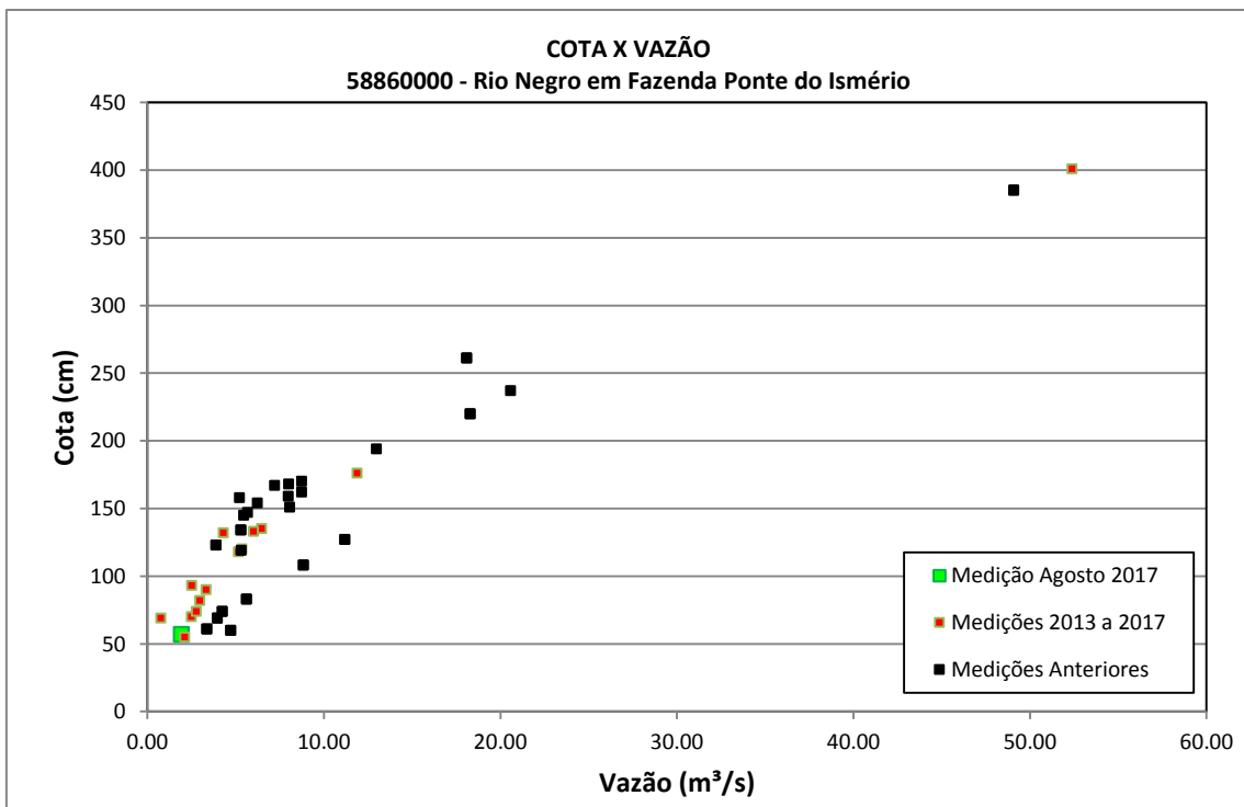
Figura 15 – Gráfico Cota x Vazão na estação Fazenda Ponte do Ismério
