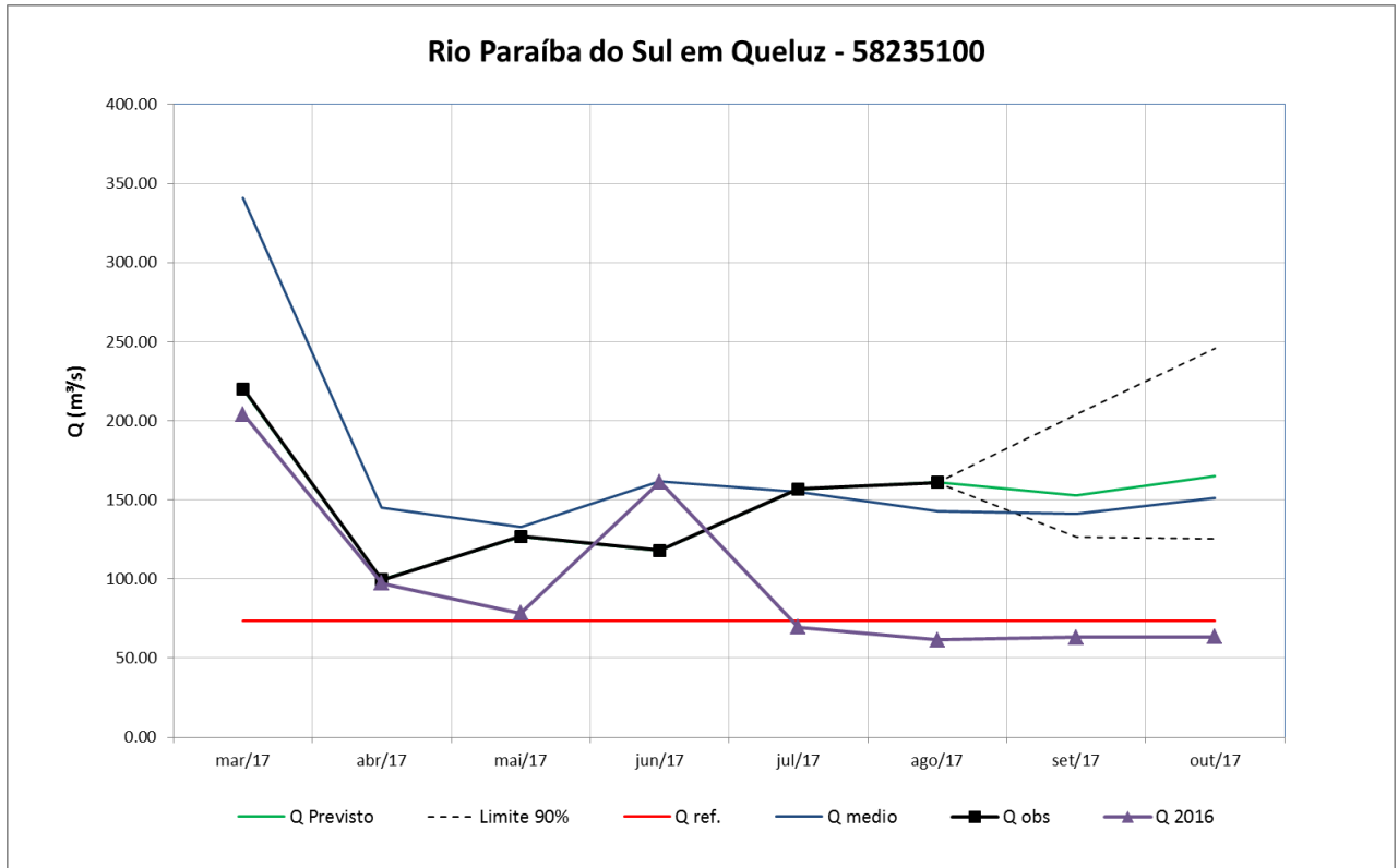
Figura 36 – Prognóstico de vazão para a estação de Queluz
