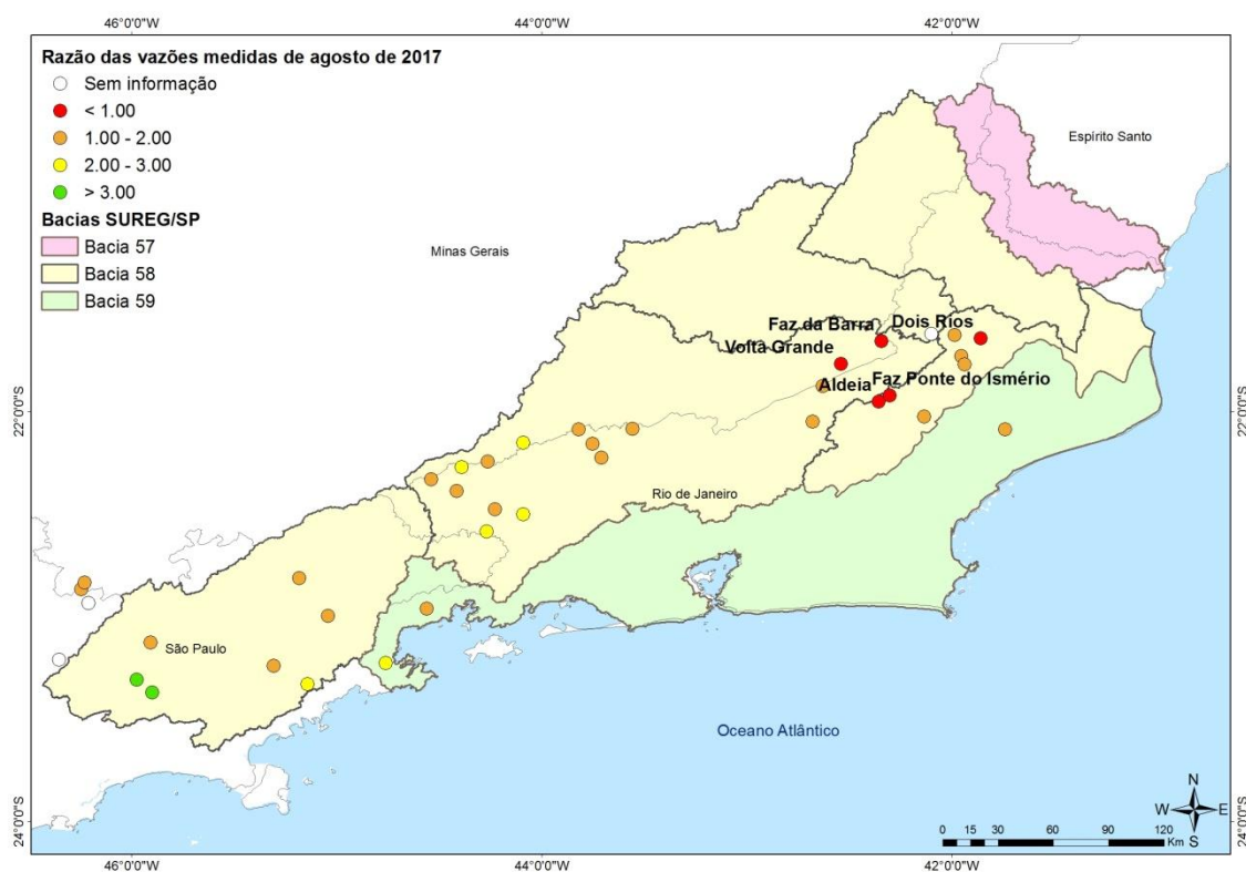
Figura 11 - Razão entre a vazão das medições de descarga líquida realizadas em agosto de 2017 e a vazão mínima histórica medida até 2013
