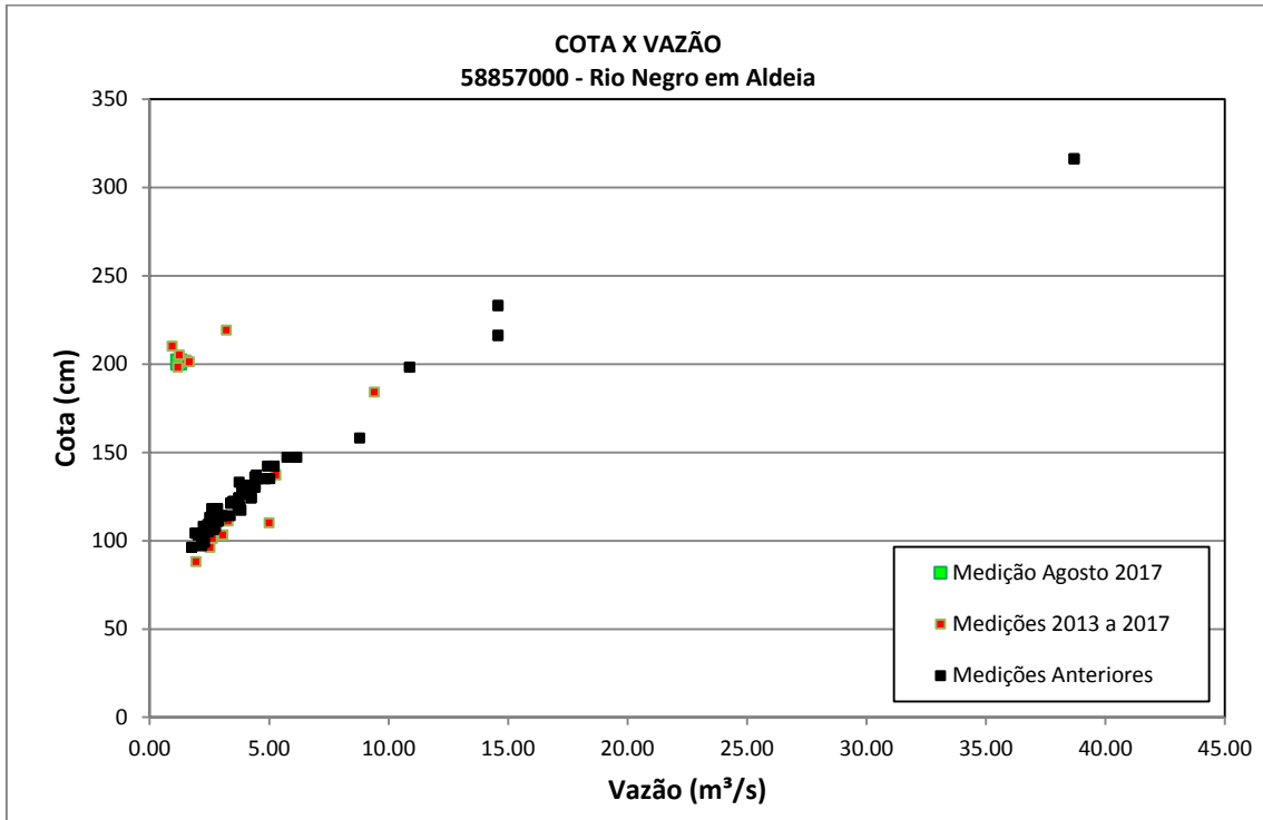
Figura 14 – Gráfico Cota x Vazão na estação Aldeia
