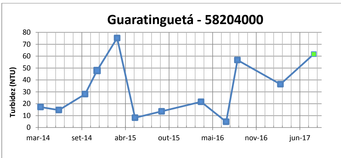
Figura 22 - Série histórica de Turbidez na estação Guaratinguetá
