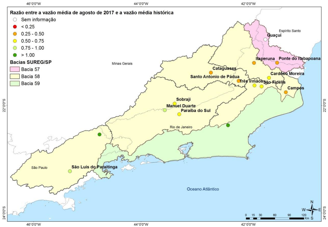
Figura 9 – Comparação entre a vazão de agosto de 2017 e a média histórica
