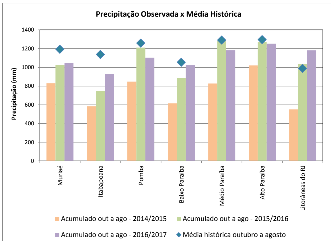
Figura 6 - Comparação entre a precipitação média histórica de outubro a agosto, a precipitação acumulada de outubro de 2014 a agosto de 2015, outubro de 2015 a agosto de 2016, e outubro de 2016 a agosto de 2017 nas bacias da área de atuação da SUREG/SP.
