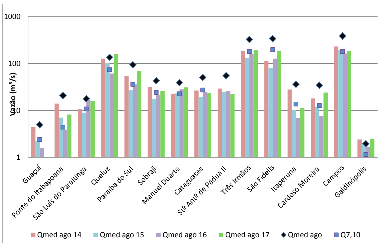
Figura 8 – Comparação entre a vazão média de agosto de 2014, 2015, 2016 e 2017, média histórica de agosto e vazão de referência Q_{7,10} nas estações indicadoras.
