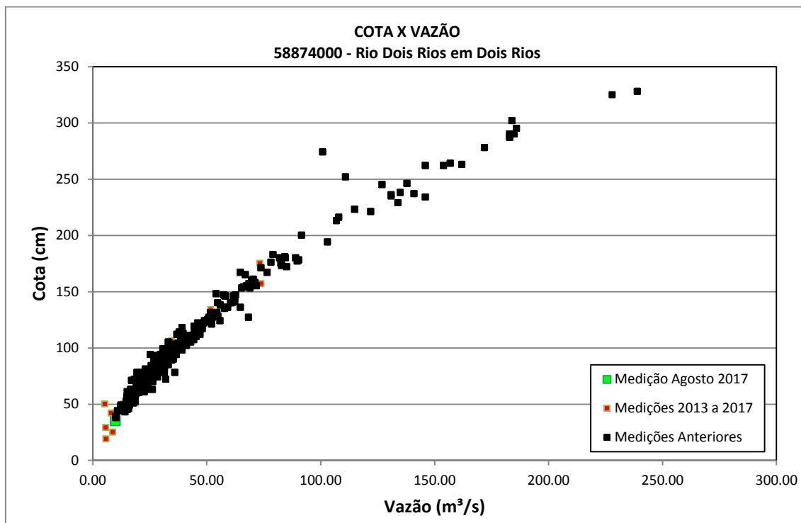
Figura 16 – Gráfico Cota x Vazão na estação Dois Rios
