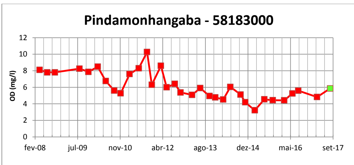
Figura 21 - Série histórica de OD na estação Pindamonhangaba
