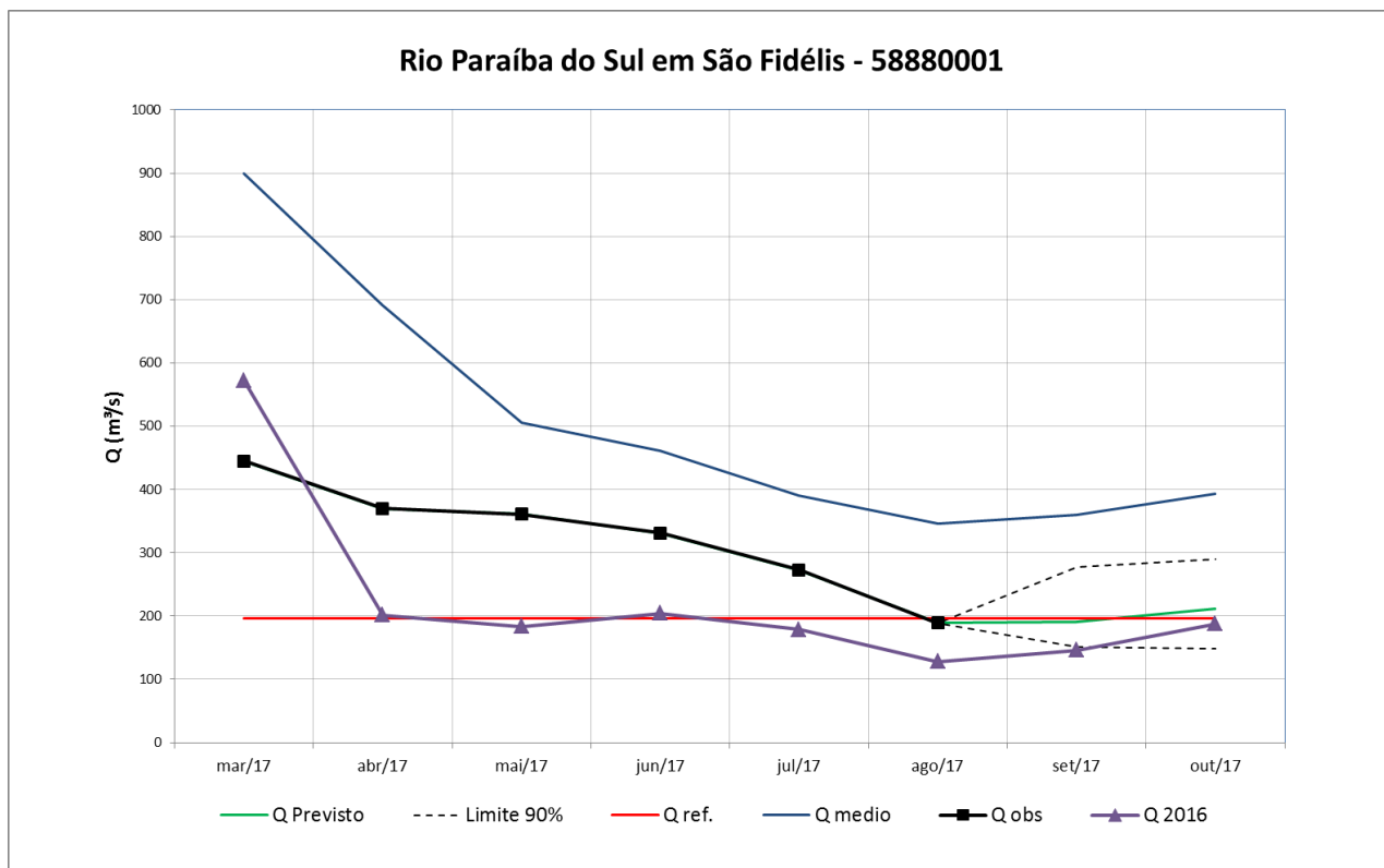
Figura 32 – Prognóstico de vazão para a estação de São Fidélis
