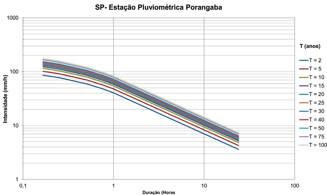
Figura 02 - Curvas intensidade-duração-frequência.
